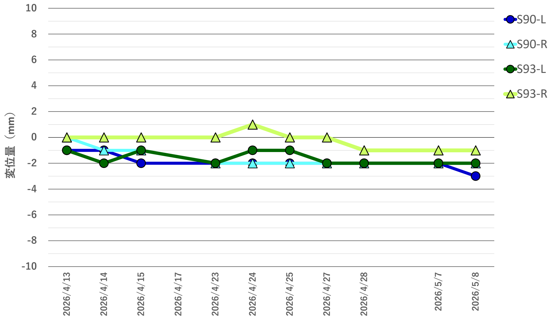
地盤変位量推移 2026年 4月 13日~2026年 5月 8日
