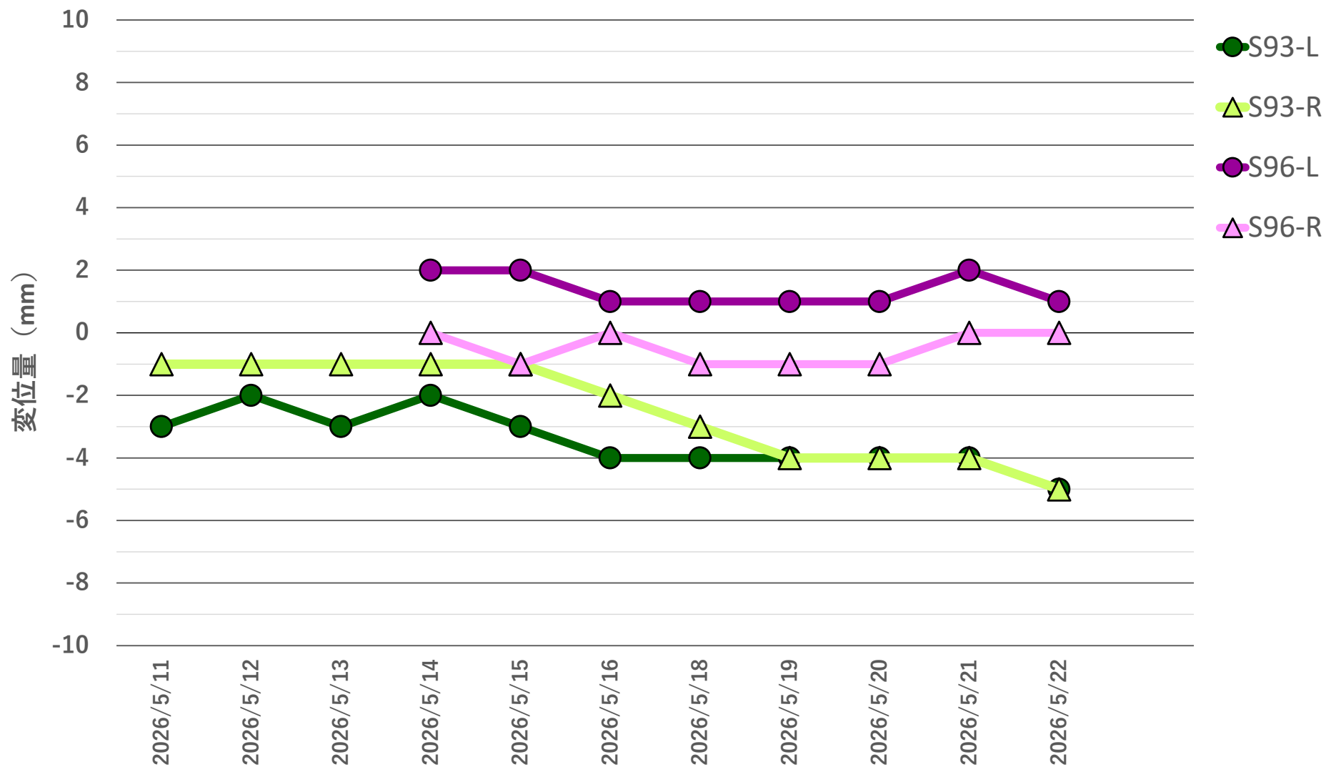
地盤変位量推移 2026年 5月 11日~2026年 5月 22日
