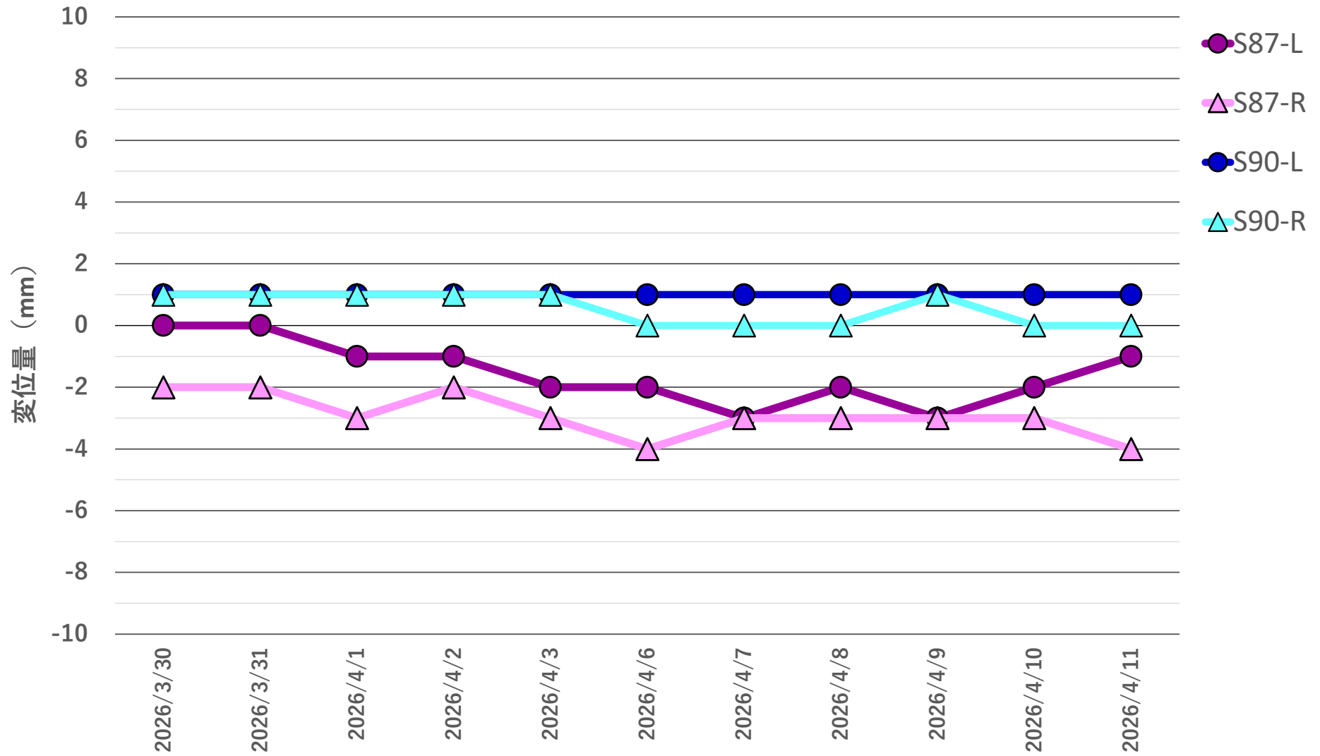
地盤変位量推移 2026年 3月 30日~2026年 4月 11日
