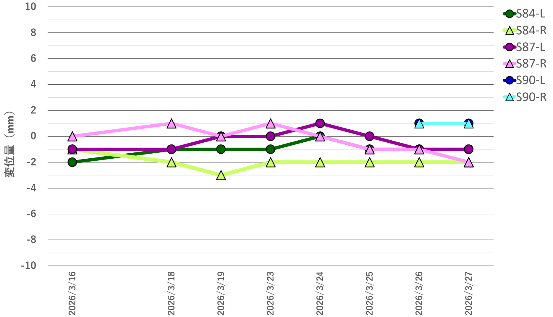
地盤変位量推移 2026年 3月 16日~2026年 3月 27日
