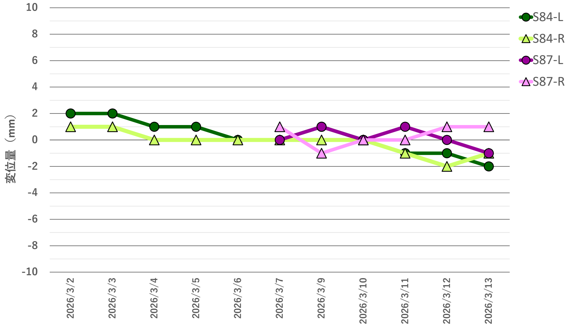
地盤変位量推移 2026年3月2日~2026年3月13日
