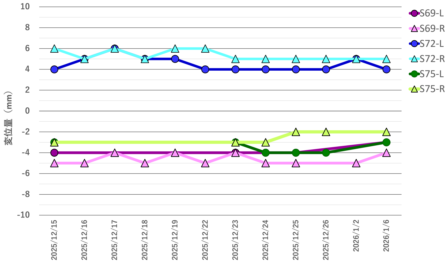
地盤変位量推移 2025年12月15日～2026年1月6日
