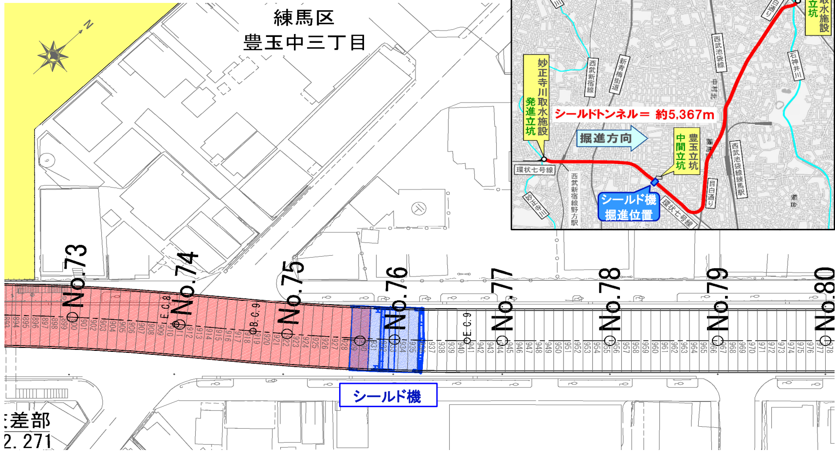
1/ 23（金）シールド機 現状位置図
