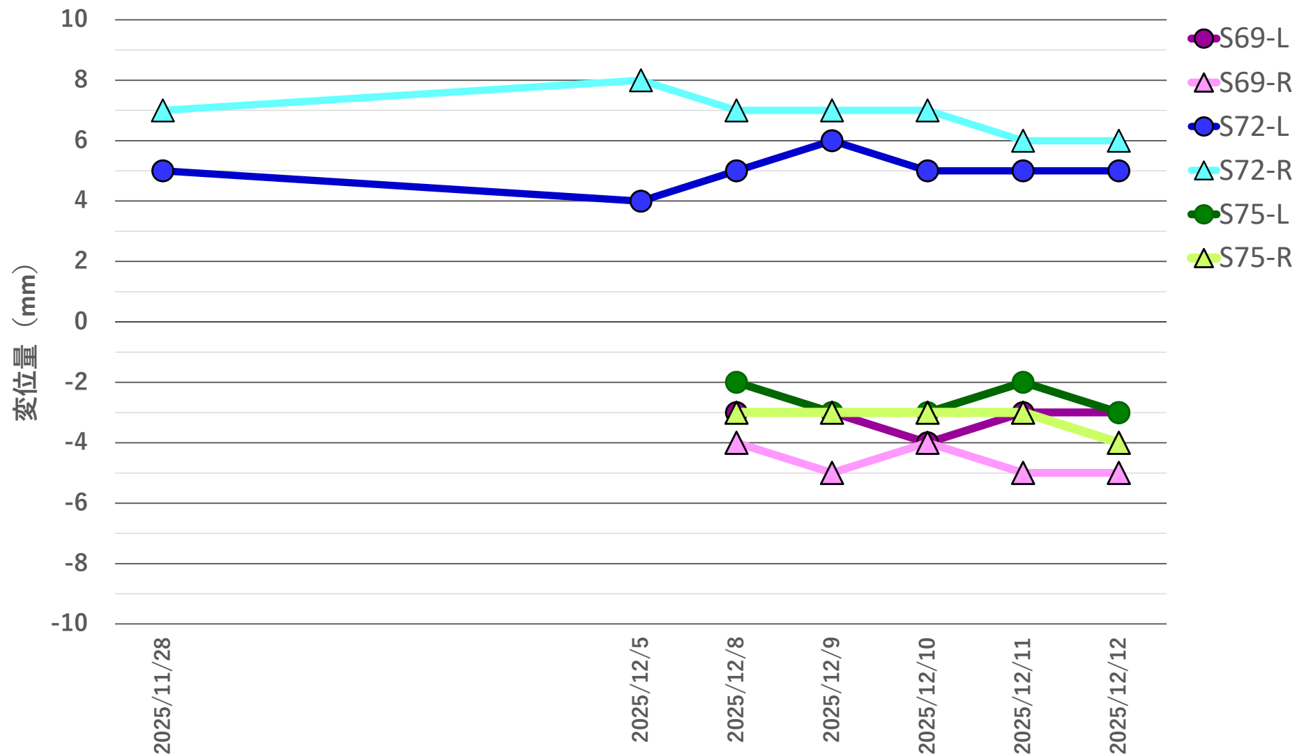
地盤変位量推移 2025年11月28日～2025年12月12日
