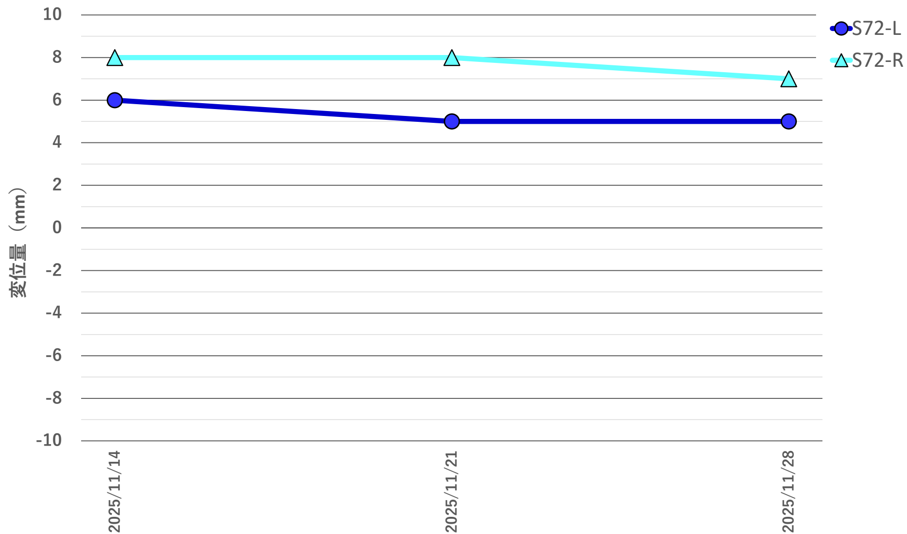
地盤変位量推移 2025年11月14日～2025年11月28日
