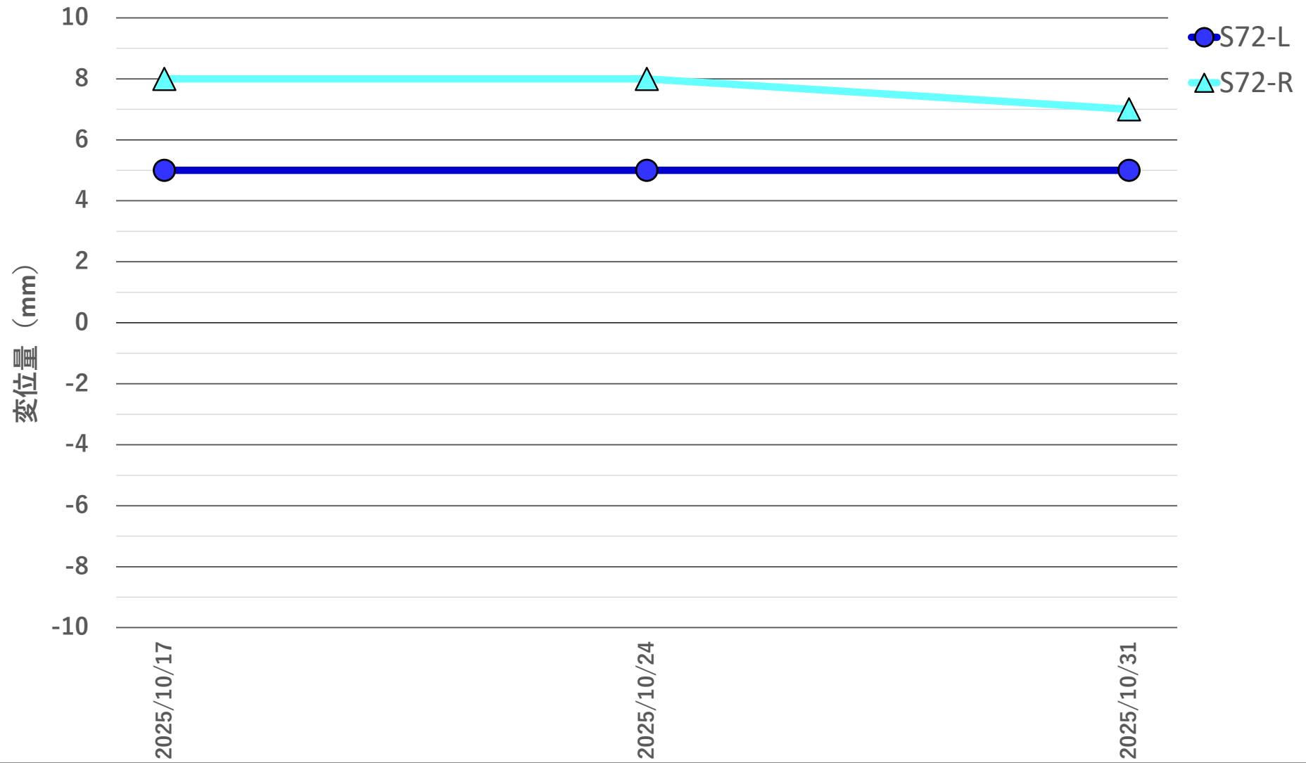
地盤変位量推移 2025年10月17日～2025年10月31日
