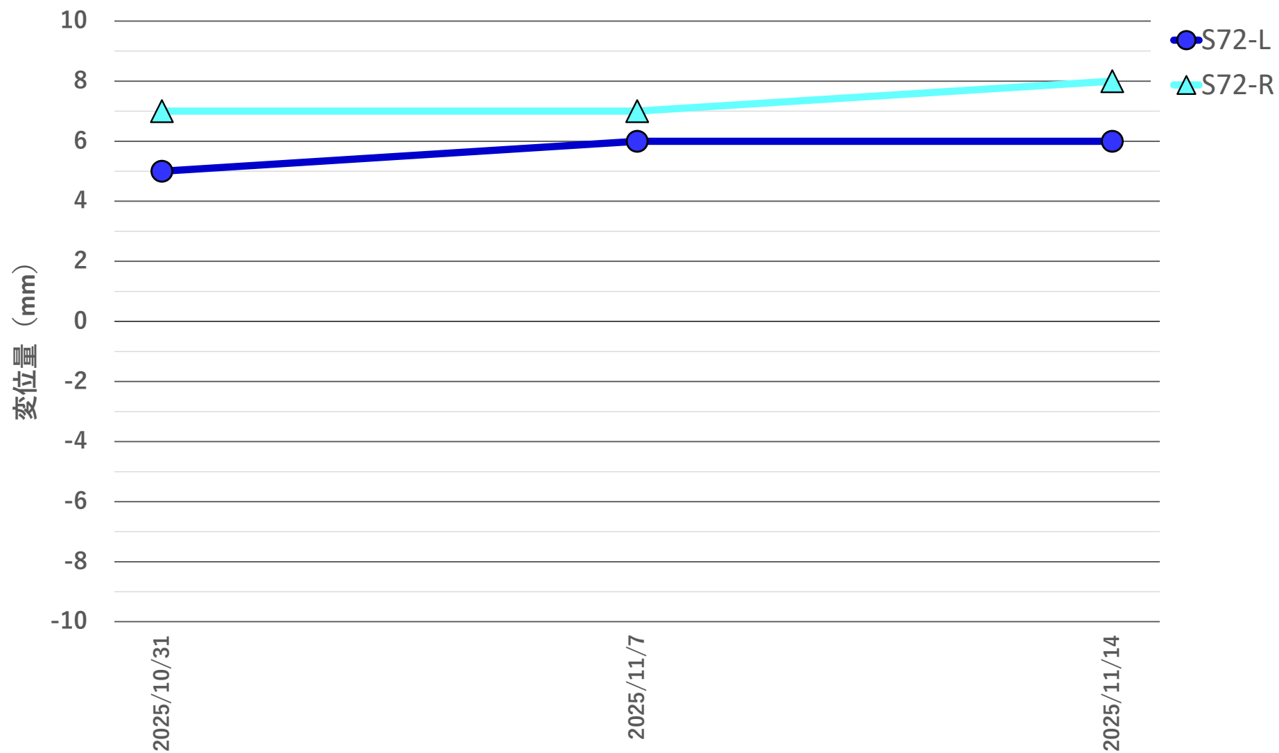
地盤変位量推移 2025年10月31日～2025年11月14日
