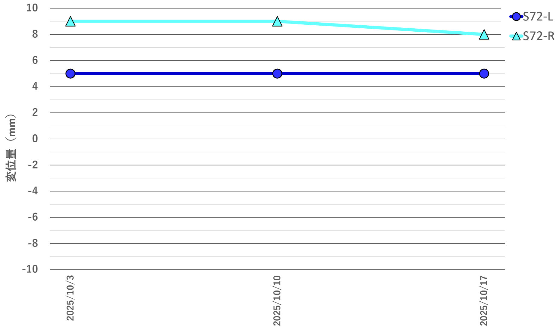
地盤変位量推移 2025年10月3日～2025年10月17日
