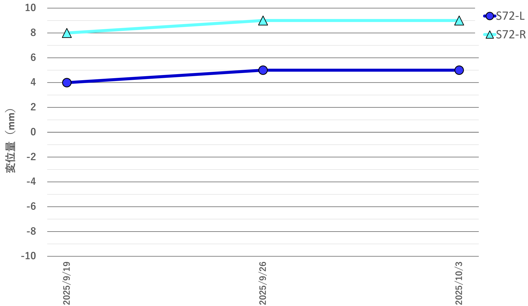
地盤変位量推移 2025年9月19日～2025年10月3日
