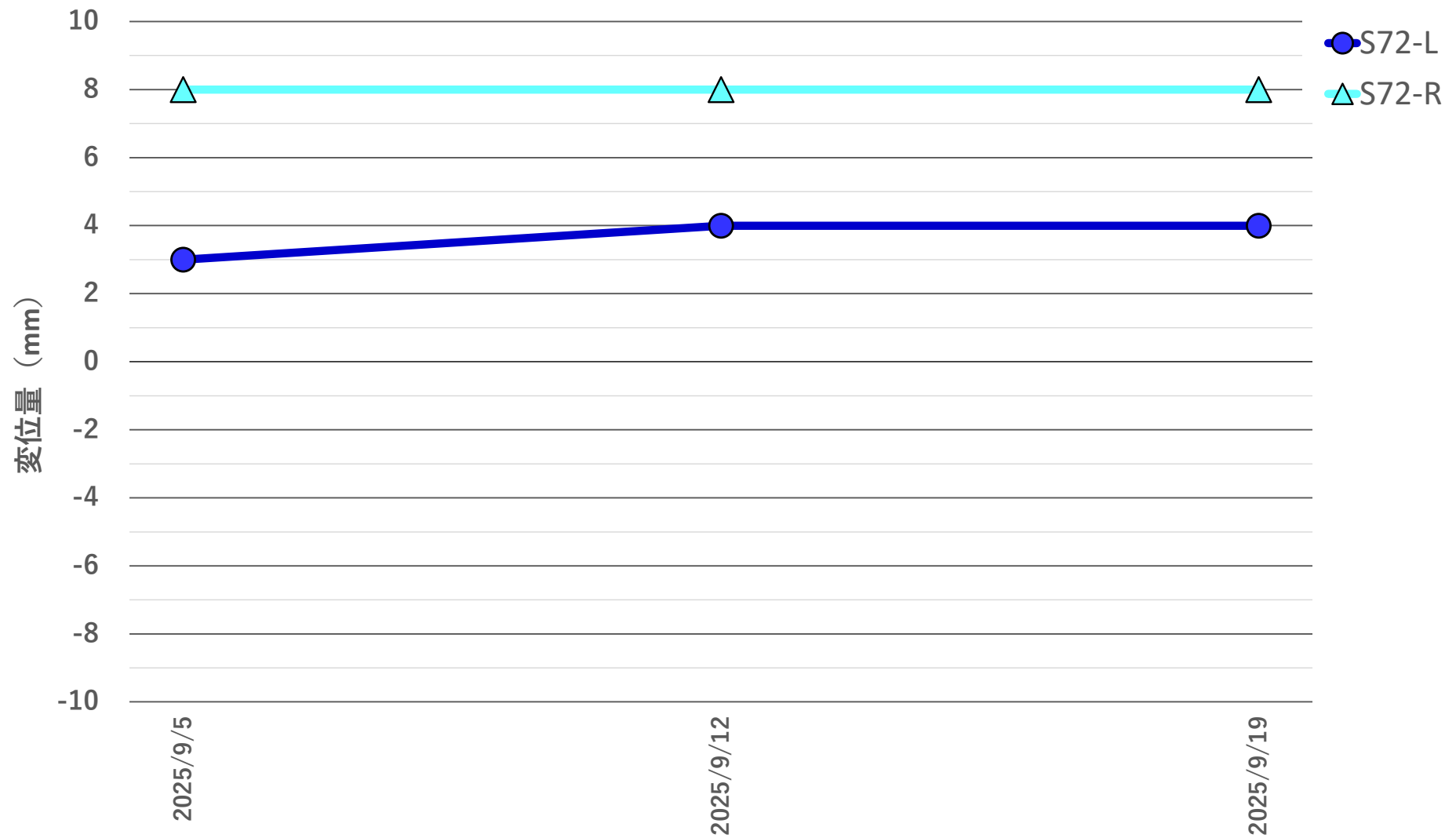
地盤変位量推移 2025年9月5日～2025年9月19日
