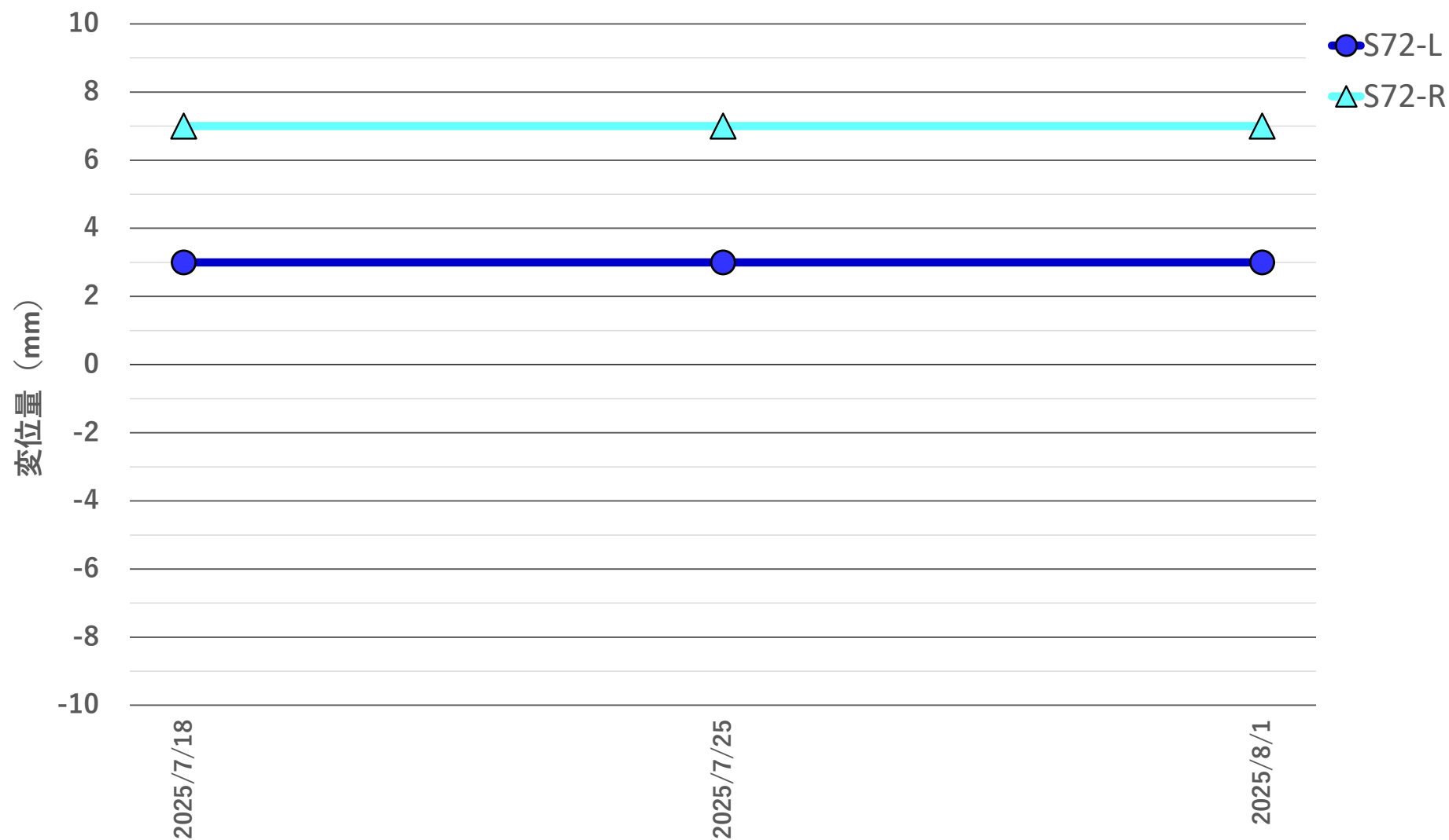
地盤変位量推移 2025年7月18日～2025年8月1日
