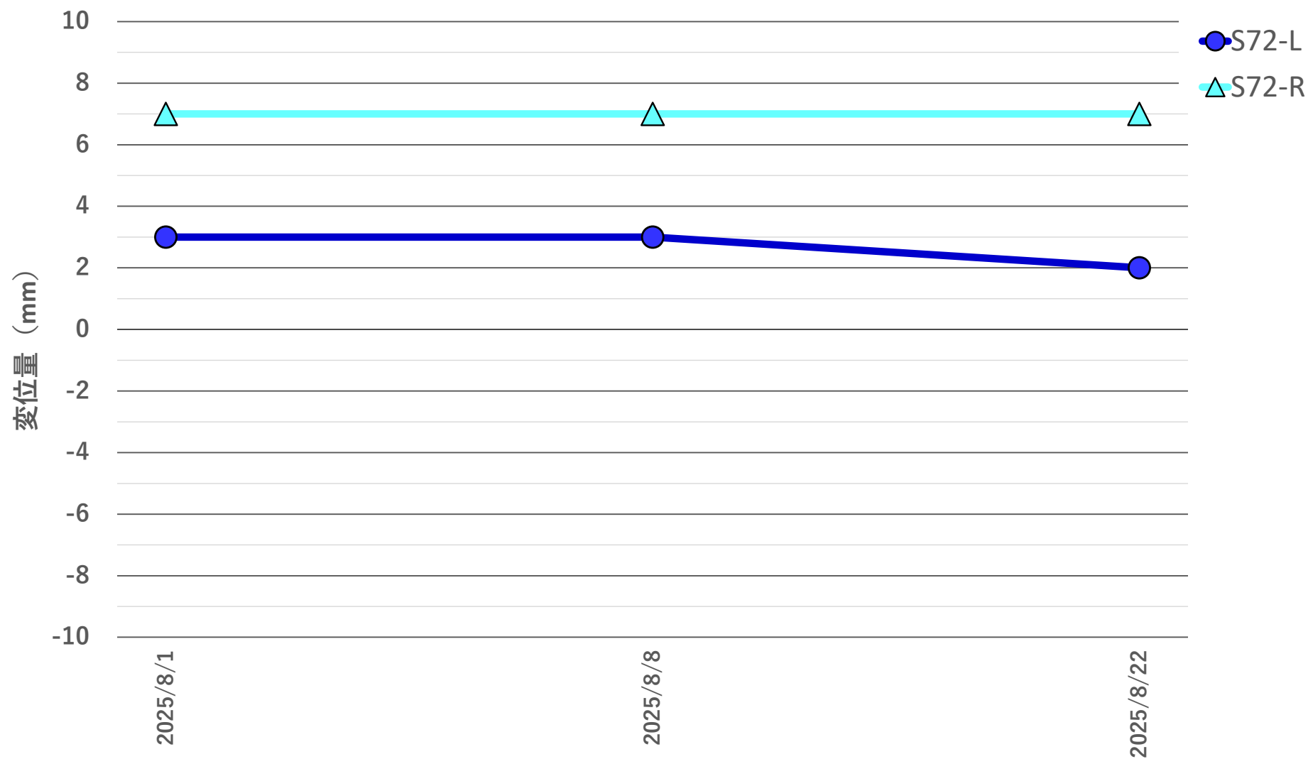
地盤変位量推移 2025年8月1日～2025年8月22日
