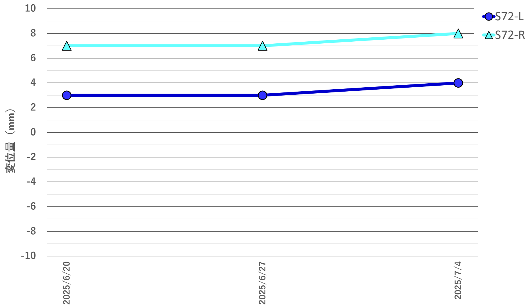
地盤変位量推移 2025年6月20日～2025年7月4日
