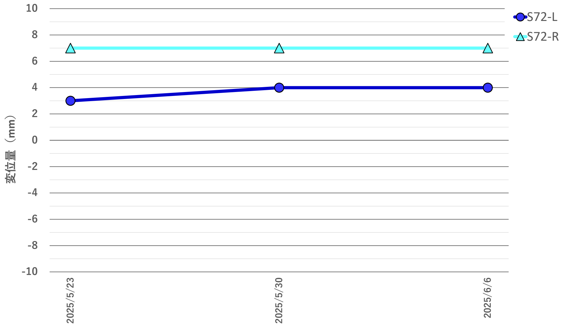
地盤変位量推移 2025年5月23日～2025年6月6日
