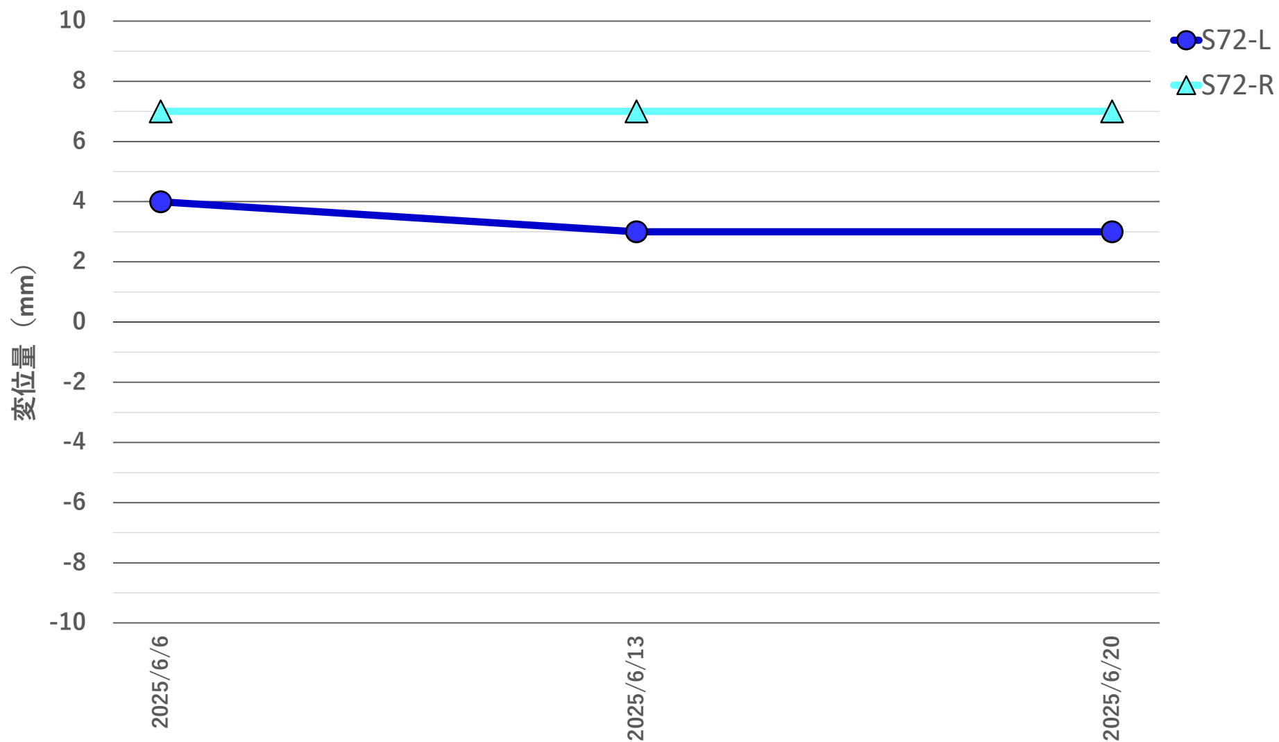
地盤変位量推移 2025年6月6日～2025年6月20日
