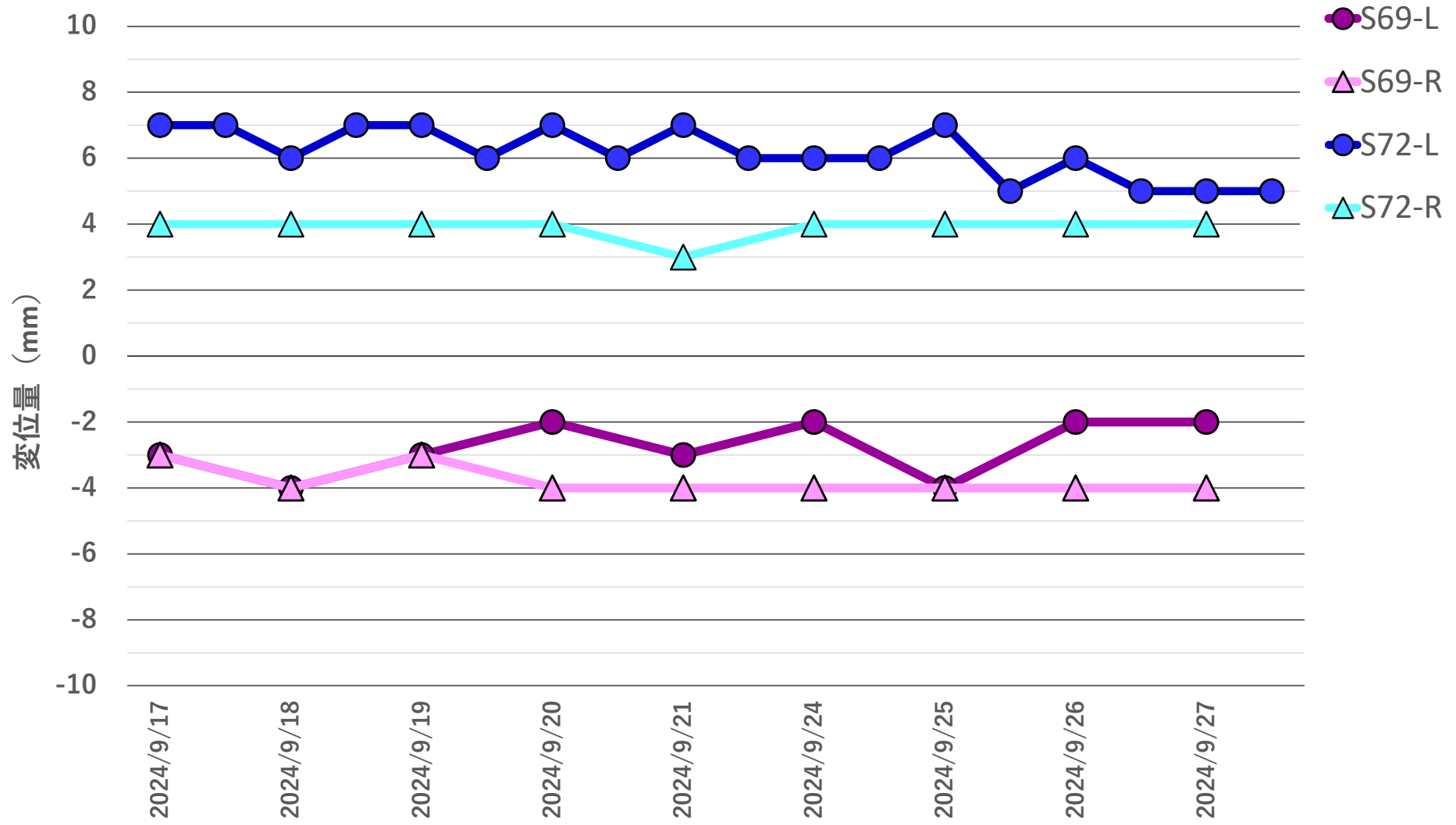
地盤変位量推移 2024年9月17日~2024年9月27日
