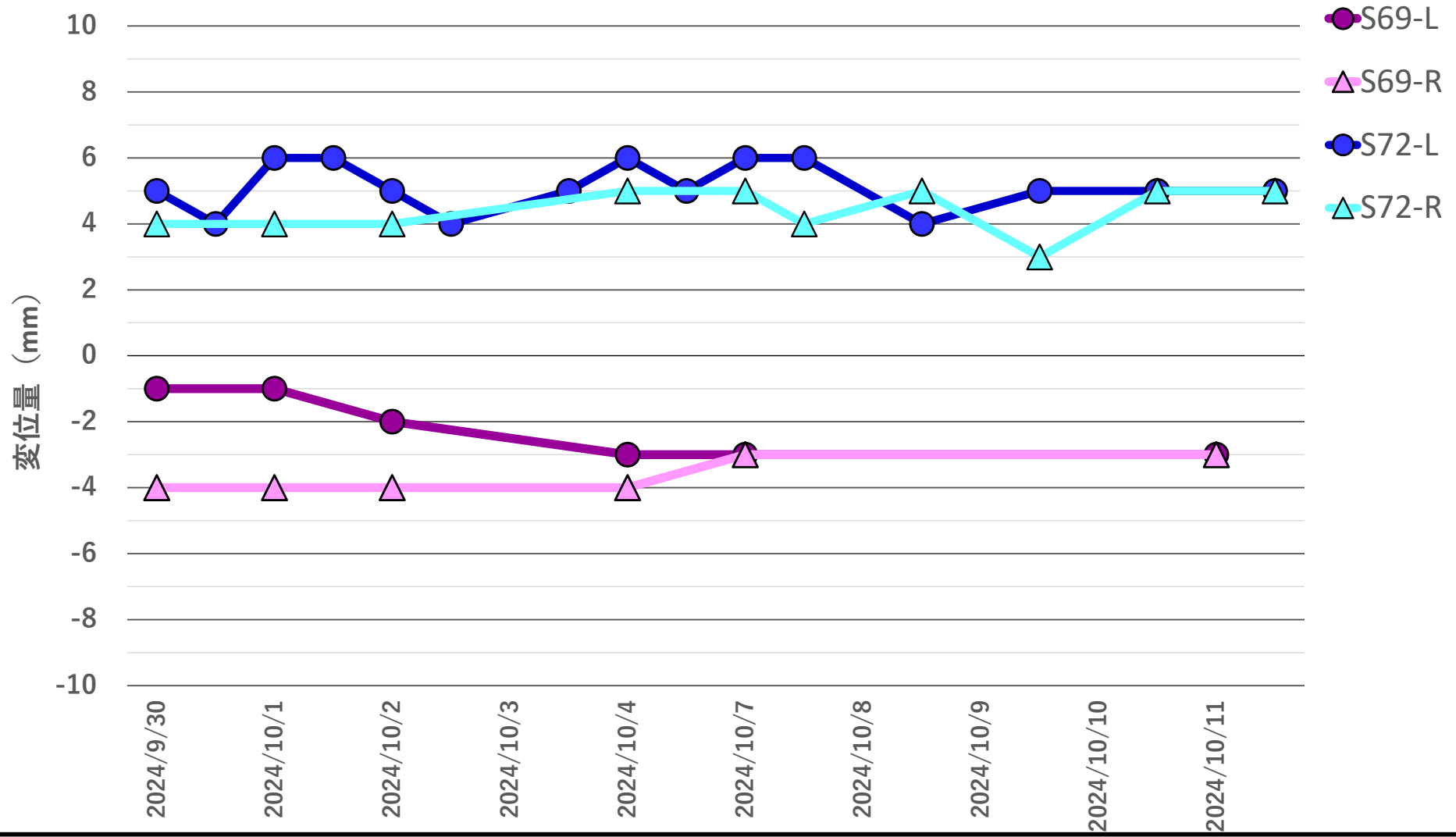
地盤変位量推移 2024年9月30日~2024年10月11日
