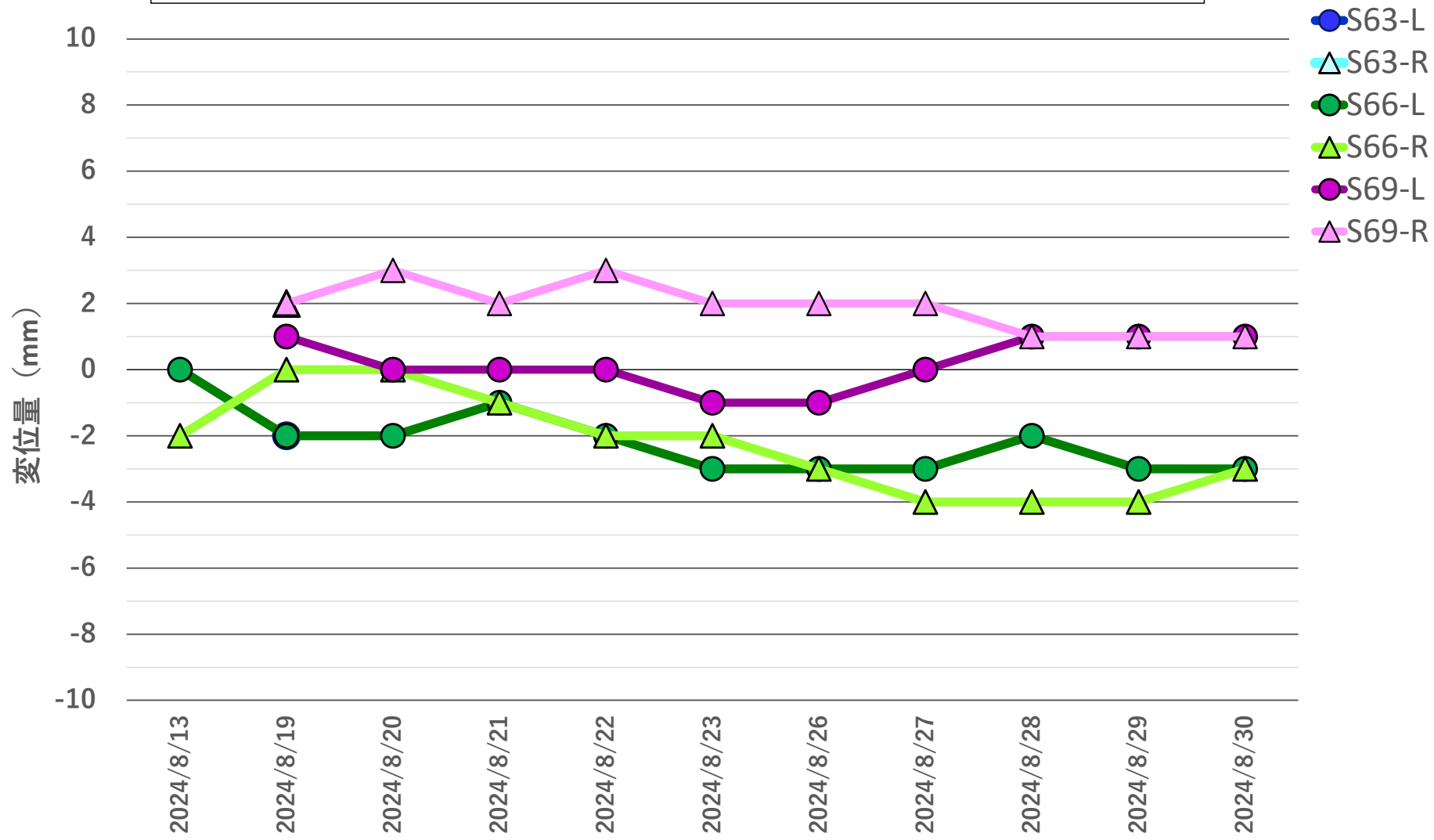
地盤変位量推移 2024年8月13日~2024年8月30日
