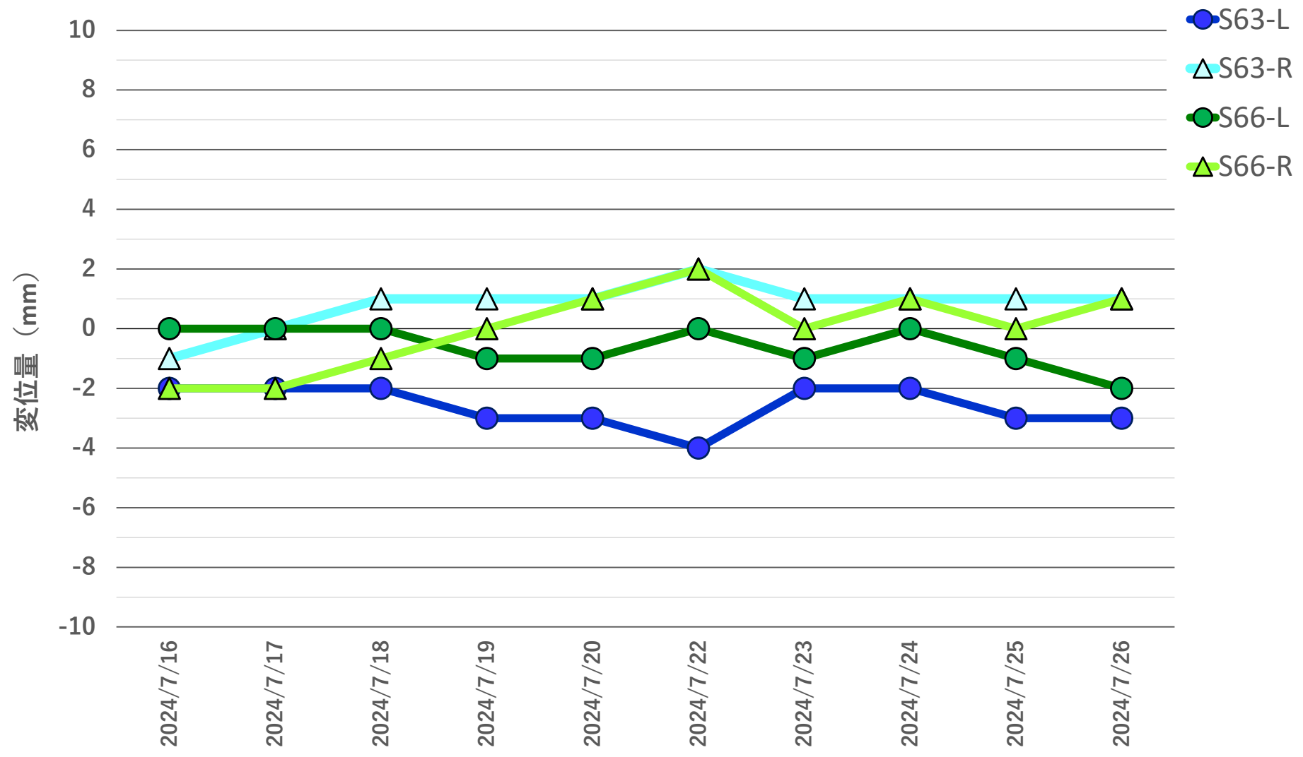
地盤変位量推移 2024年7月16日~2024年7月26日
