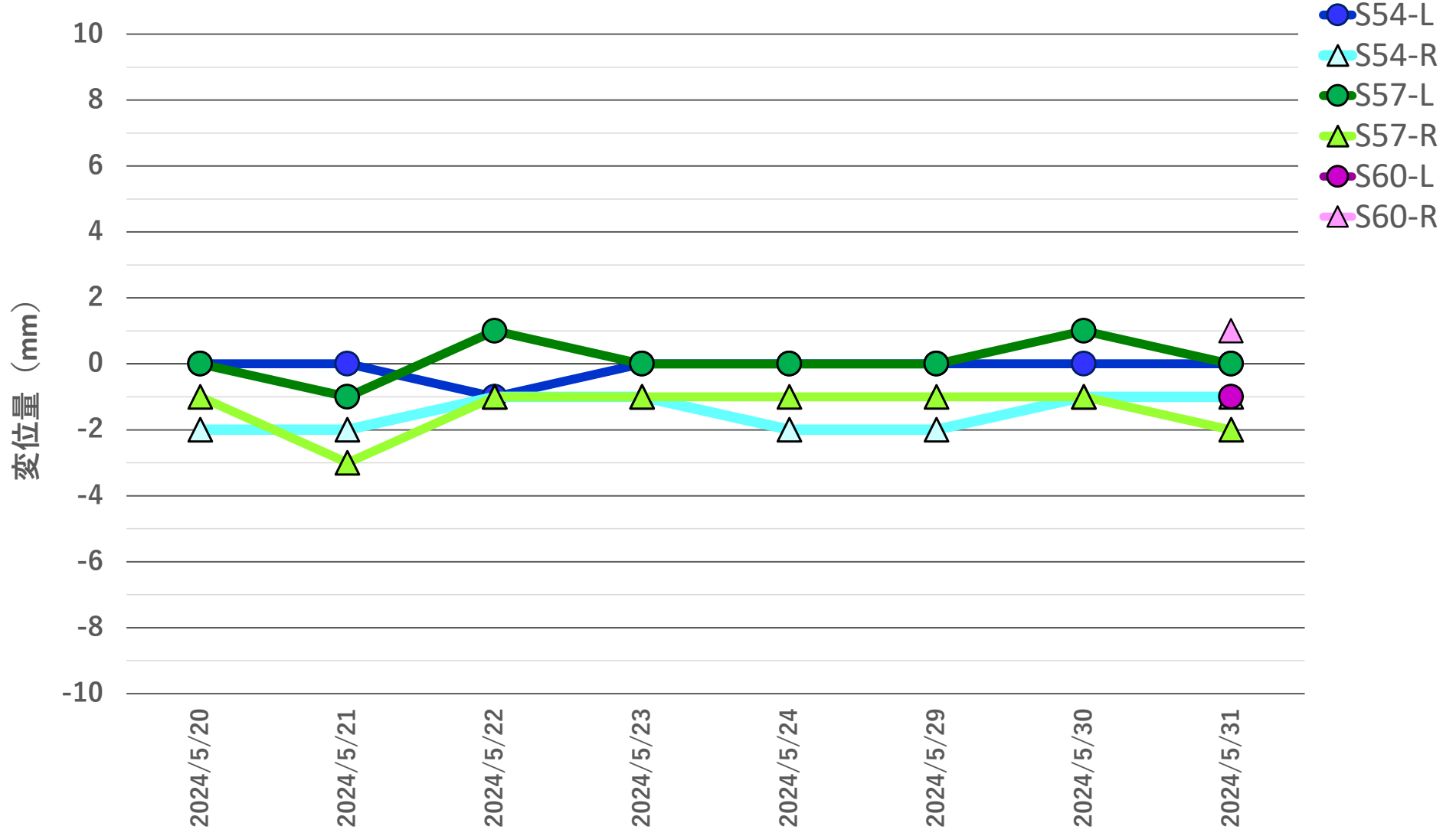
地盤変位量推移 2024年5月20日~2024年5月31日
