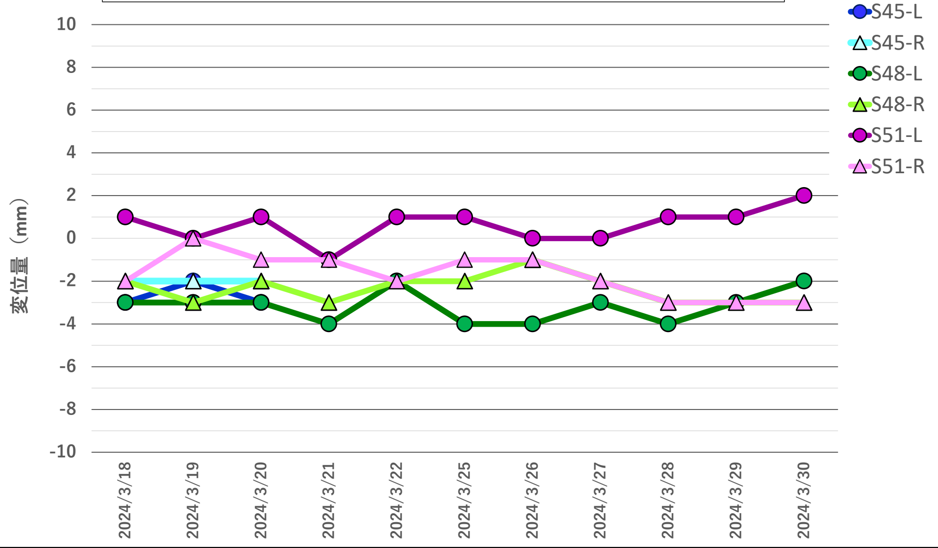
地盤変位量推移 2024年3月18日~2024年3月30日
