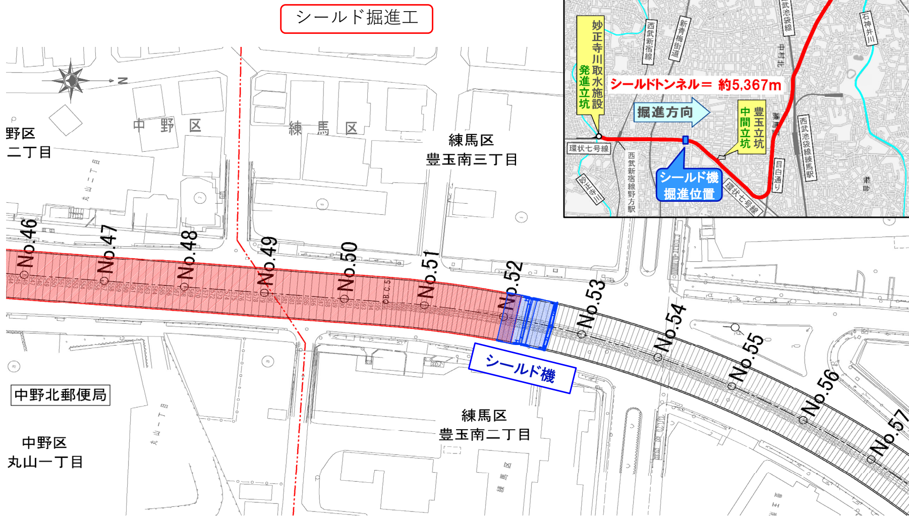
4 / 19 (金) シールド機 現状位置図
