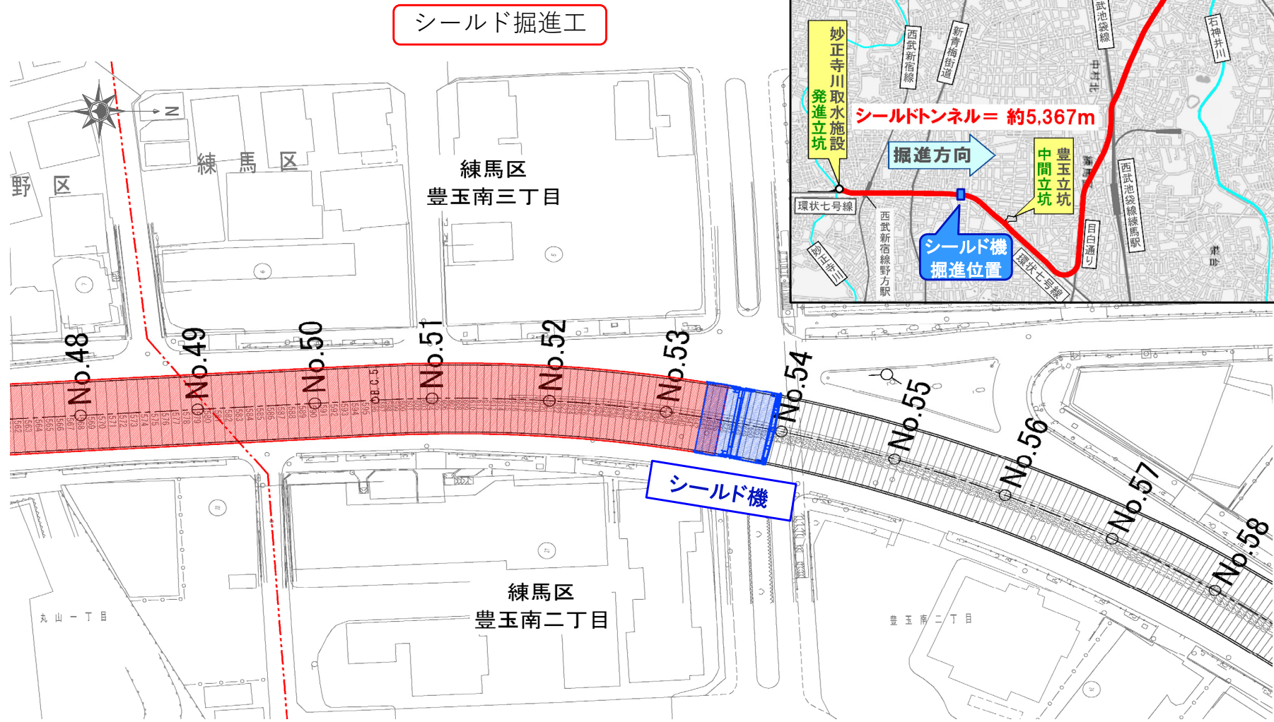
4 / 26 (金) シールド機 現状位置図
