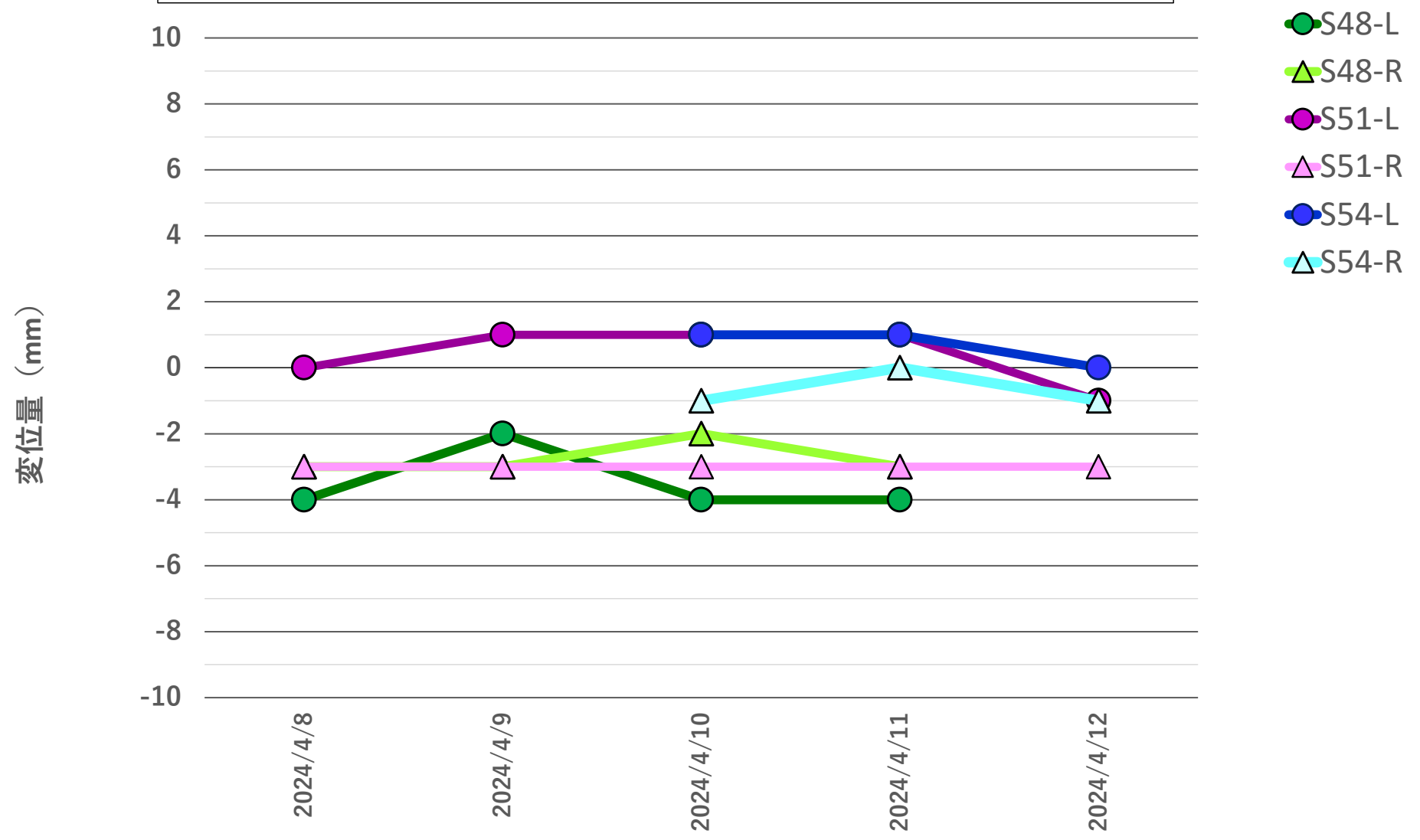
地盤変位量推移 2024年4月8日~2024年4月12日
