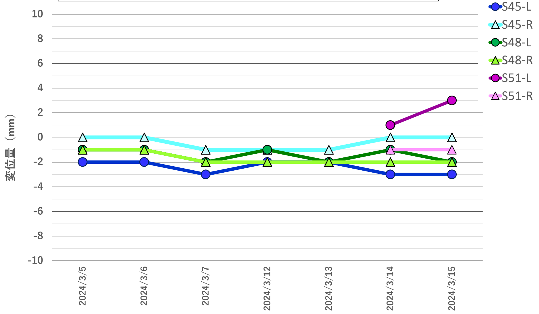
地盤変位量推移 2024年3月5日~2024年3月15日
