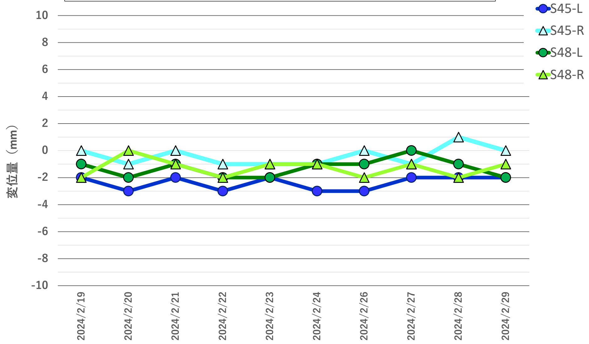
地盤変位量推移 2024年2月19日~2024年2月29日
