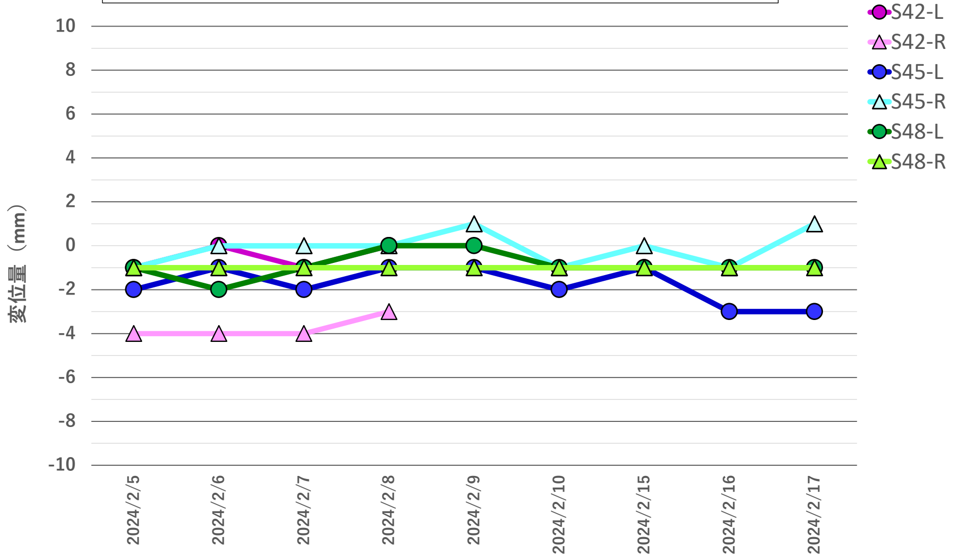
地盤変位量推移 2024年2月5日~2024年2月17日
