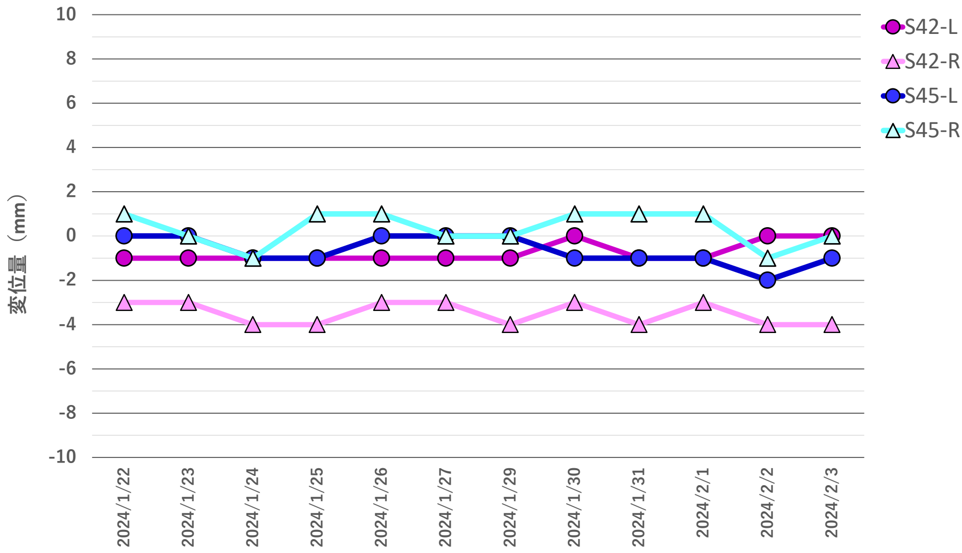
地盤変位量推移 2024年1月22日~2024年2月3日
