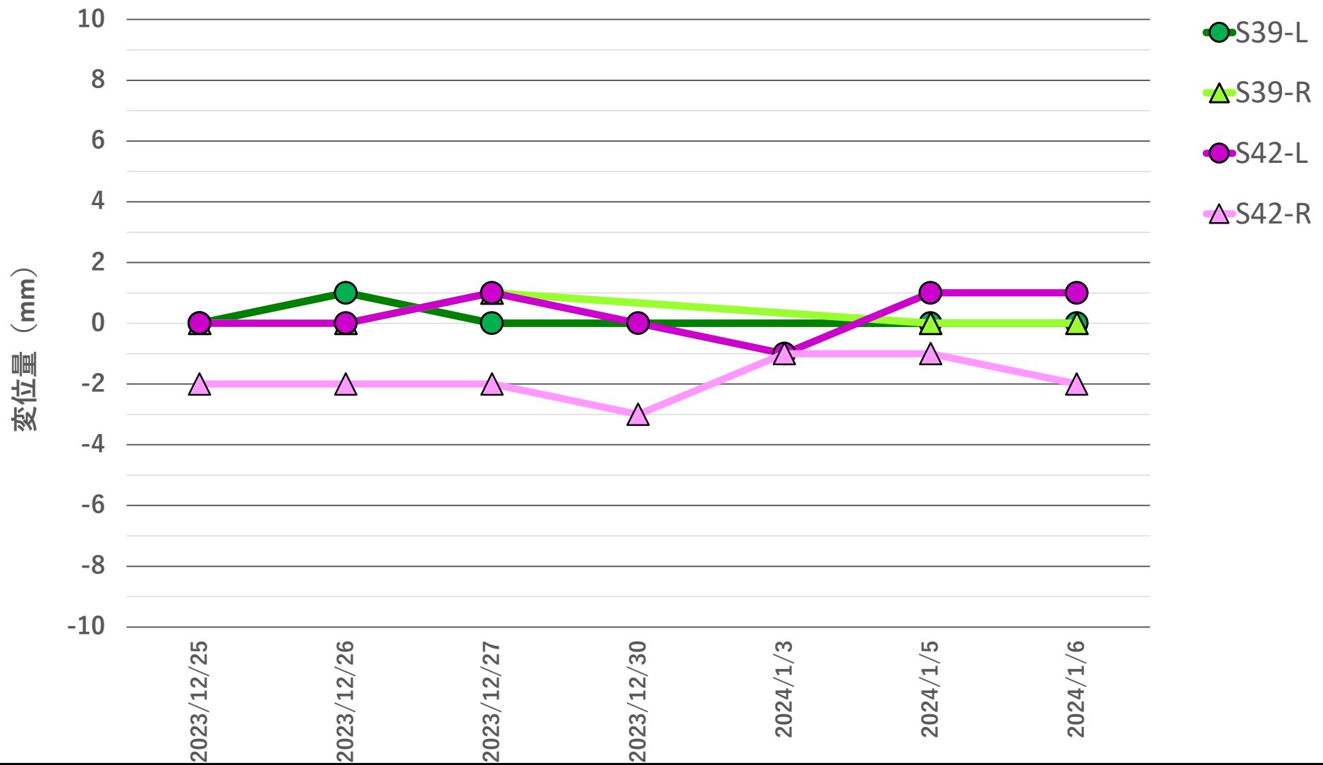
地盤変位量推移 2023年12月25日~2024年1月6日
