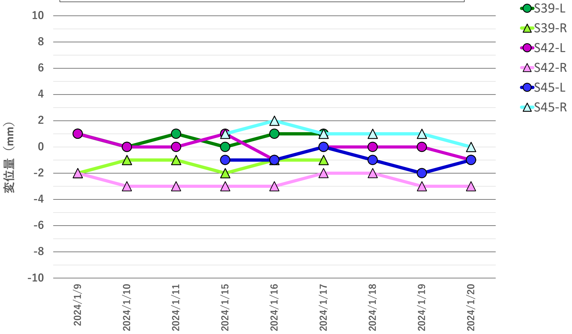
地盤変位量推移 2024年1月9日~2024年1月20日
