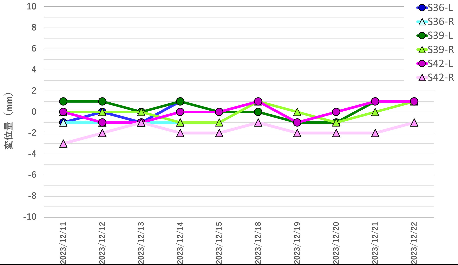
地盤変位量推移 2023年12月11日~2023年12月22日
