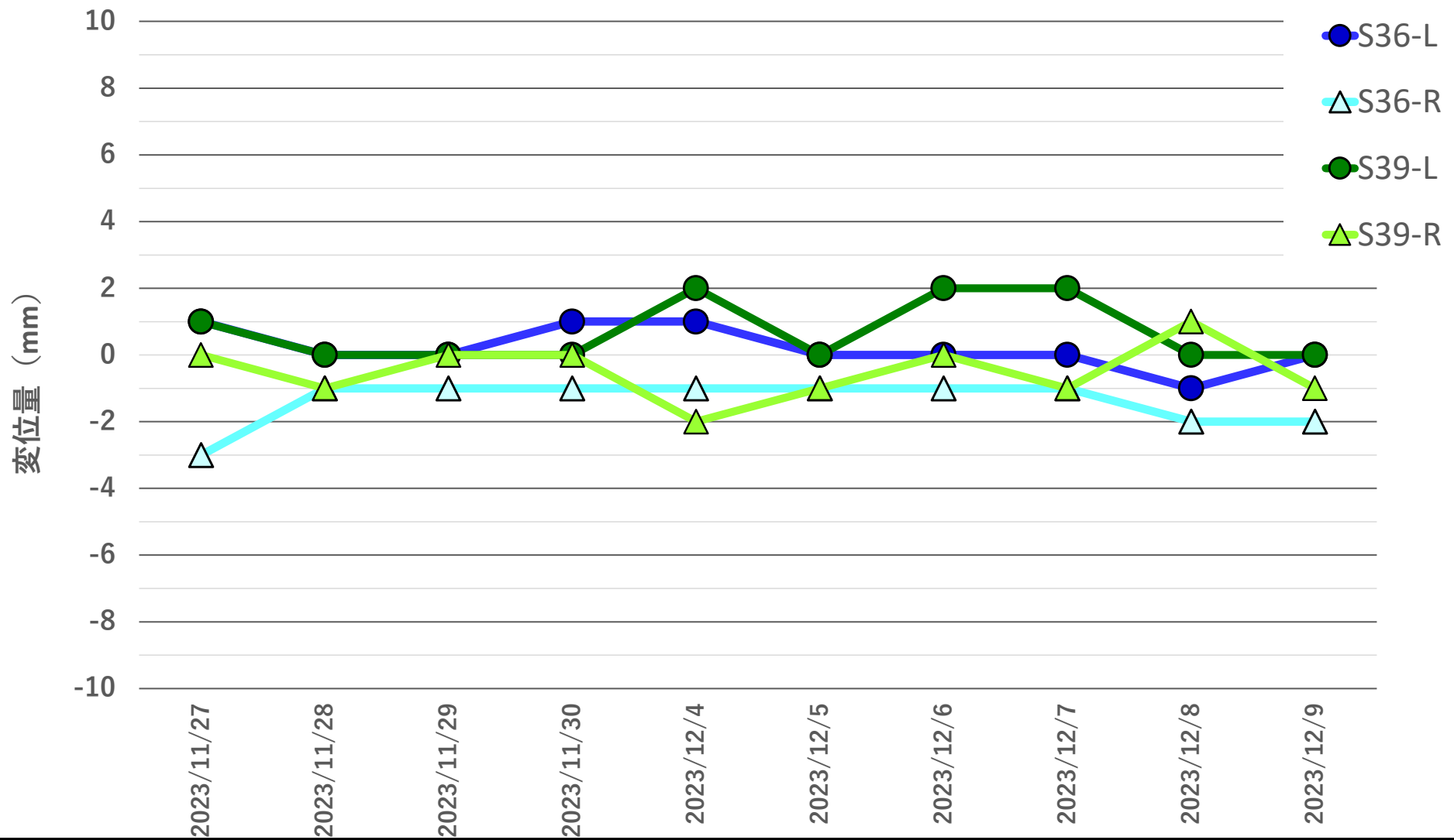
地盤変位量推移 2023年11月27日~2023年12月9日
