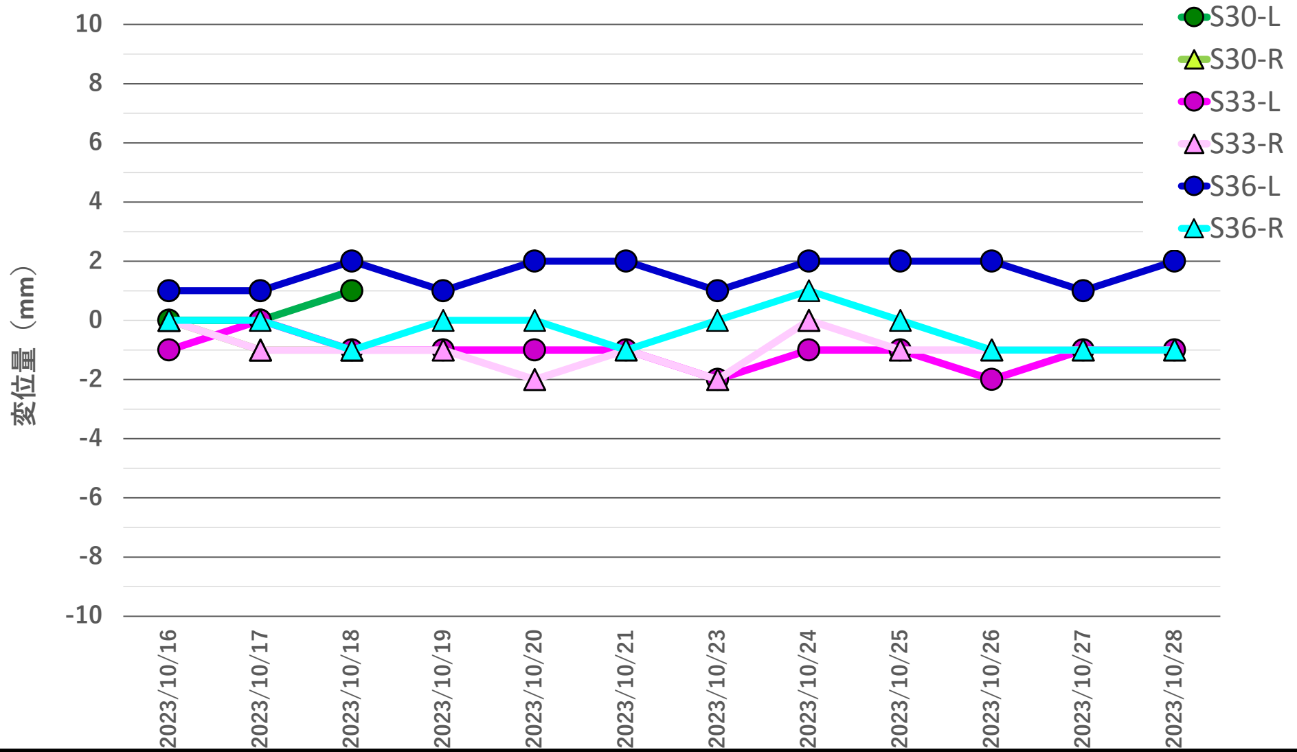
地盤変位量推移 2023年10月16日~2023年10月28日
