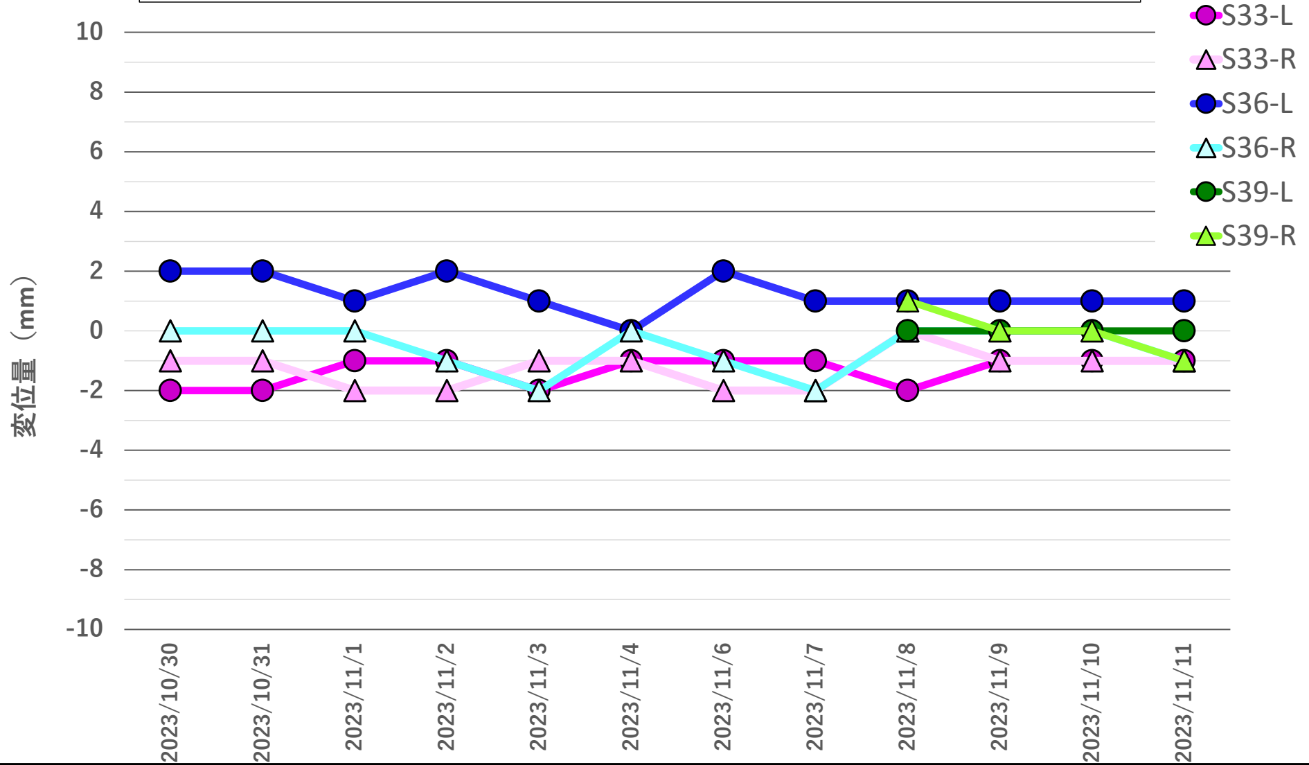
地盤変位量推移 2023年10月30日~2023年11月11日
