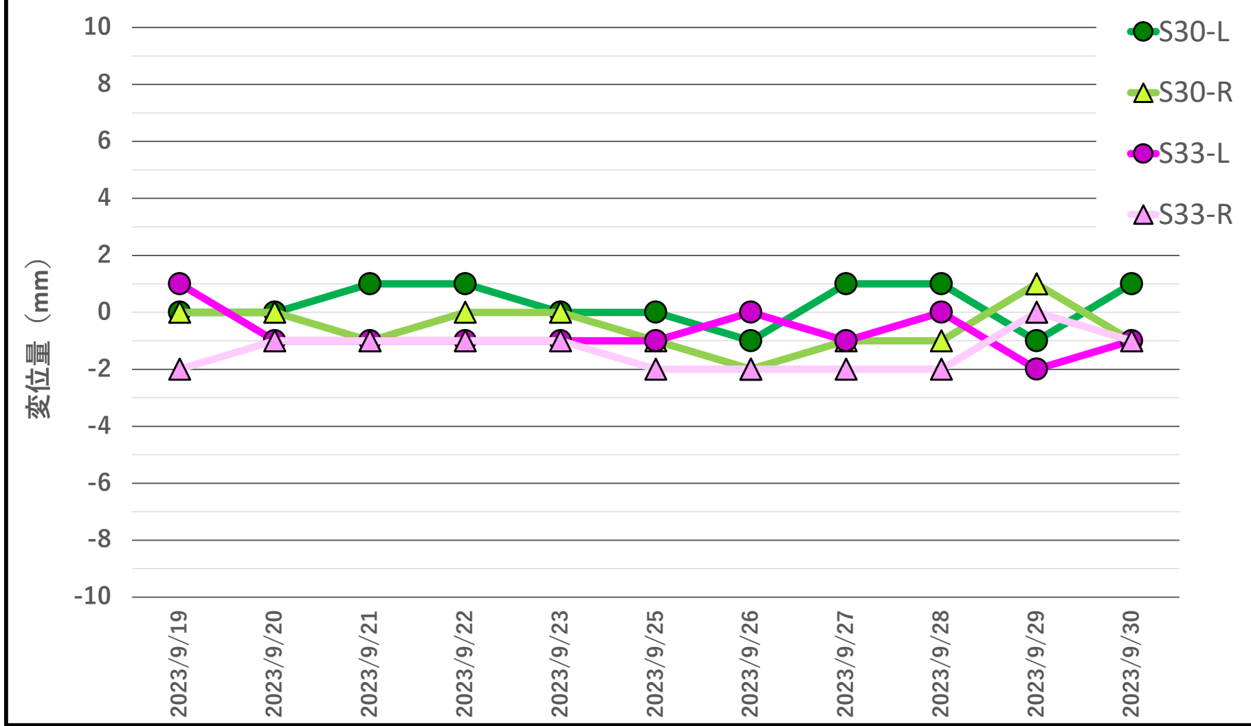
地盤変位量推移 2023年9月19日~2023年9月30日
