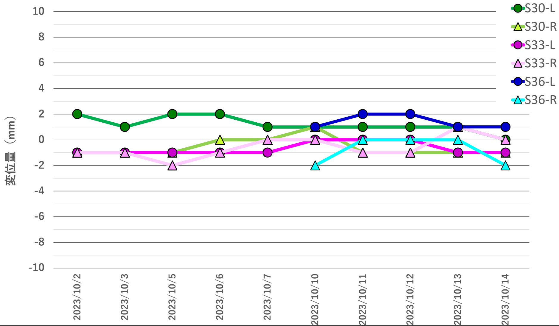
地盤変位量推移 2023年10月2日~2023年10月14日
