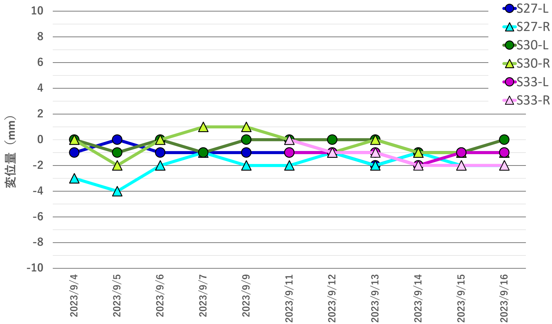
地盤変位量推移 2023年9月4日~2023年9月16日
