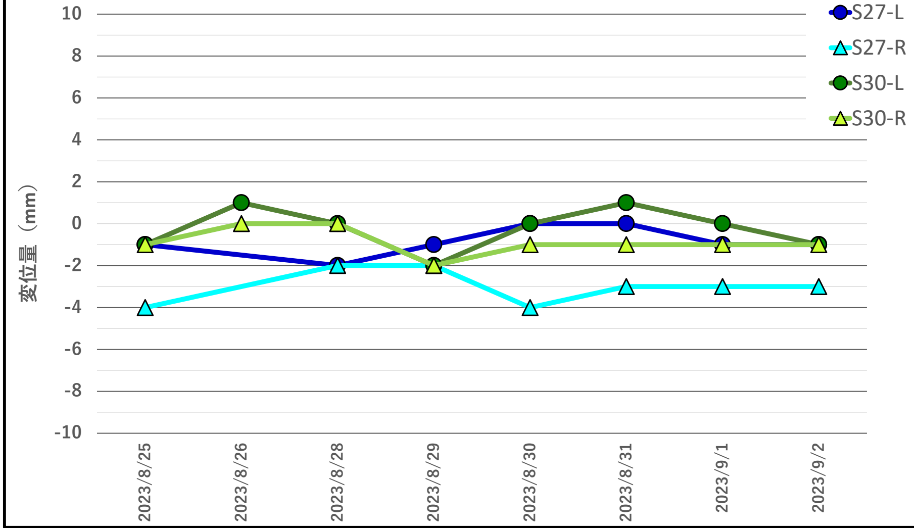
地盤変位量推移 2023年8月25日~2023年9月2日
