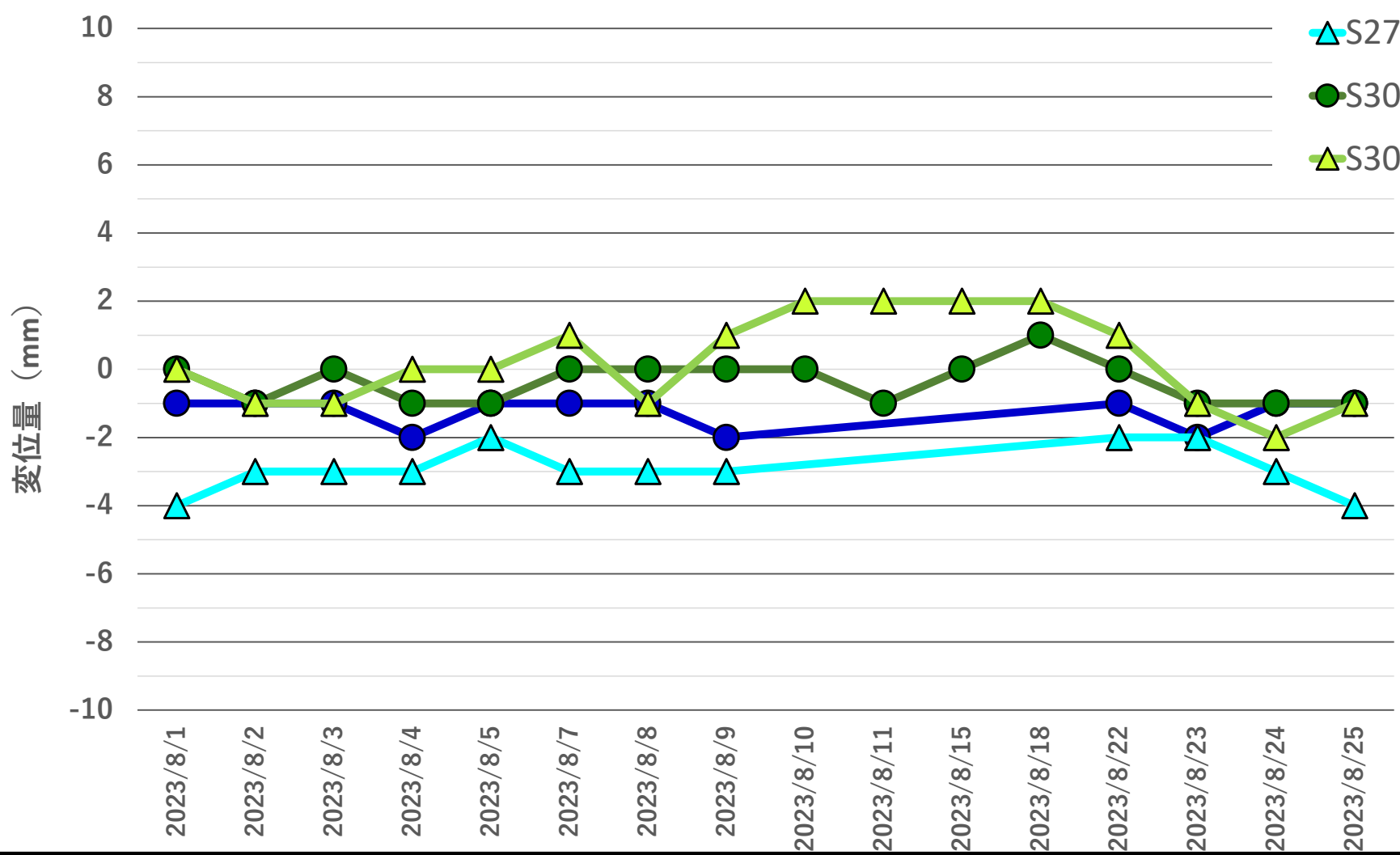
地盤変位量推移 2023年8月1日~2023年8月25日
