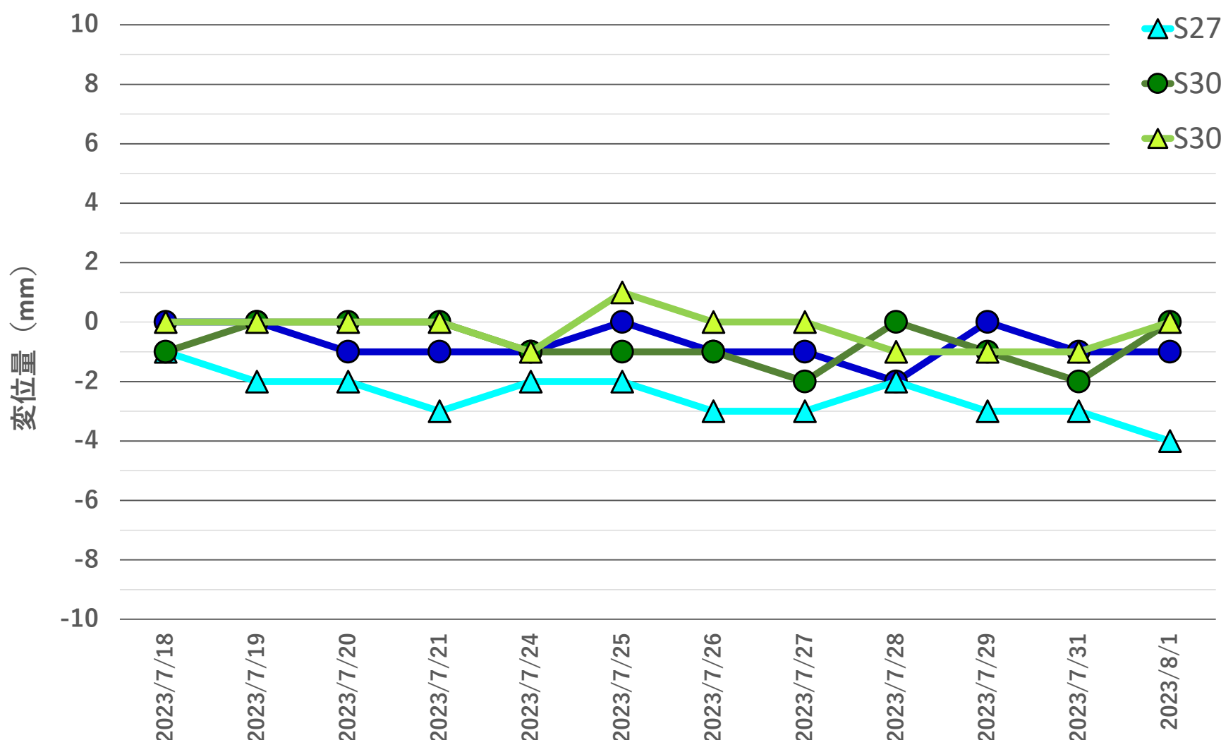
地盤変位量推移 2023年7月18日~2023年8月1日
