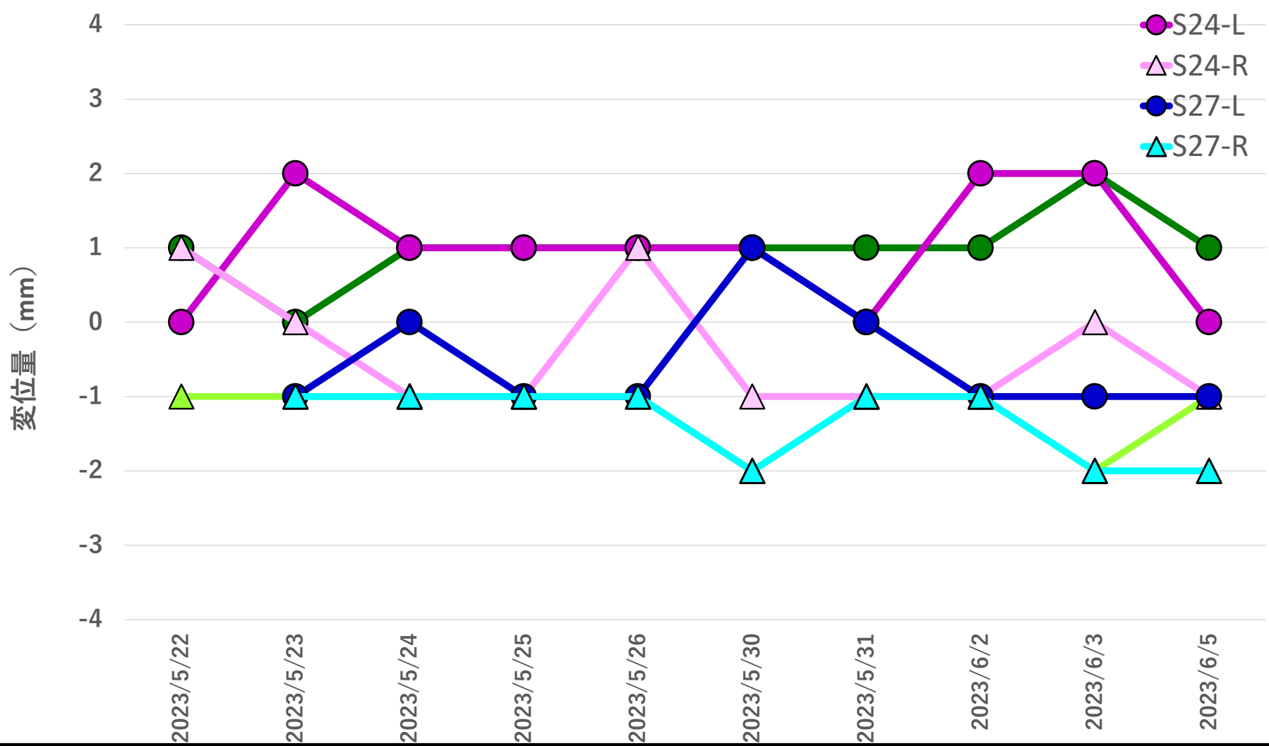
地盤変位量推移 2023年5月22日~2023年6月5日
