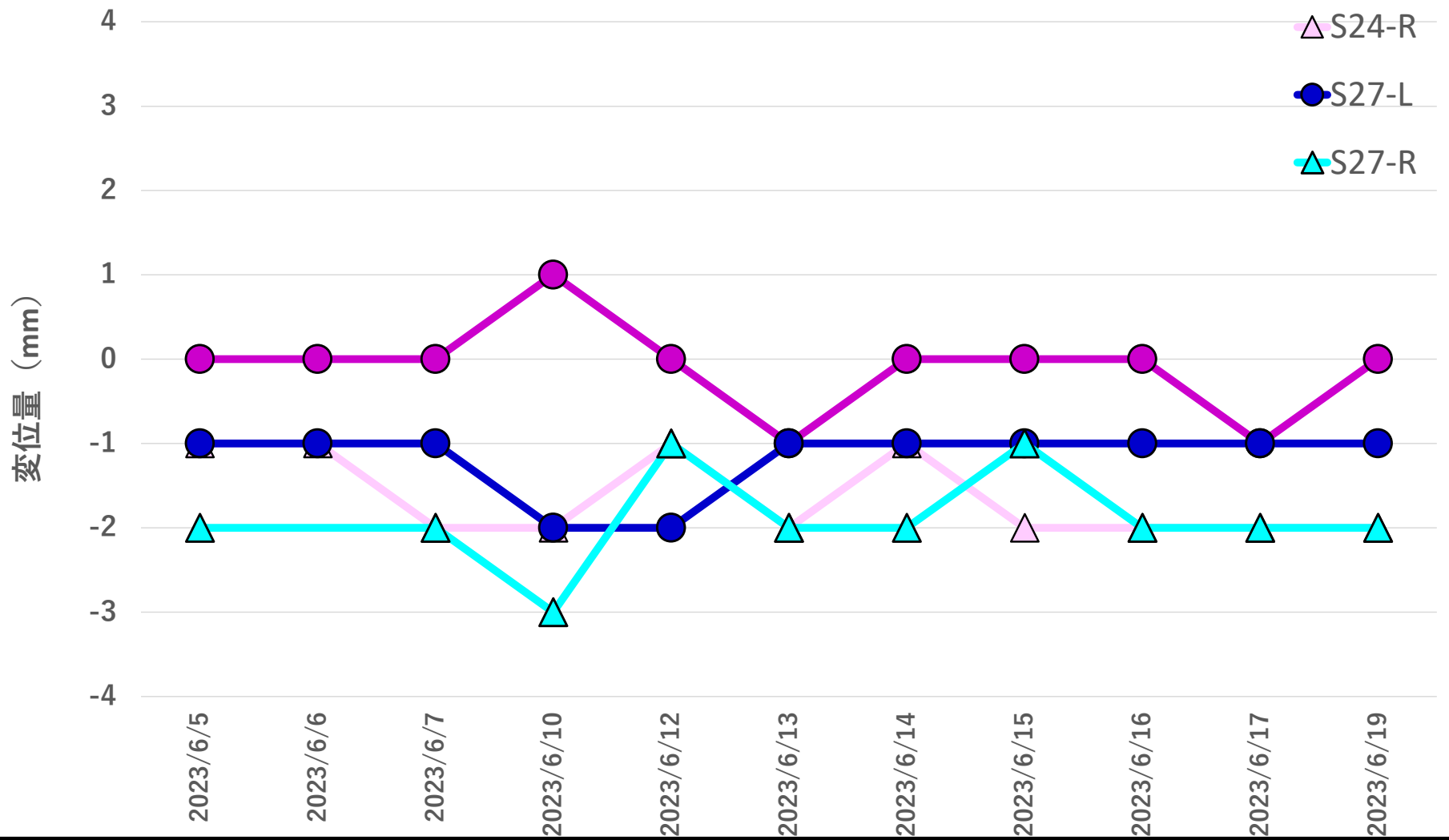
地盤変位量推移 2023年6月5日~2023年6月19日
