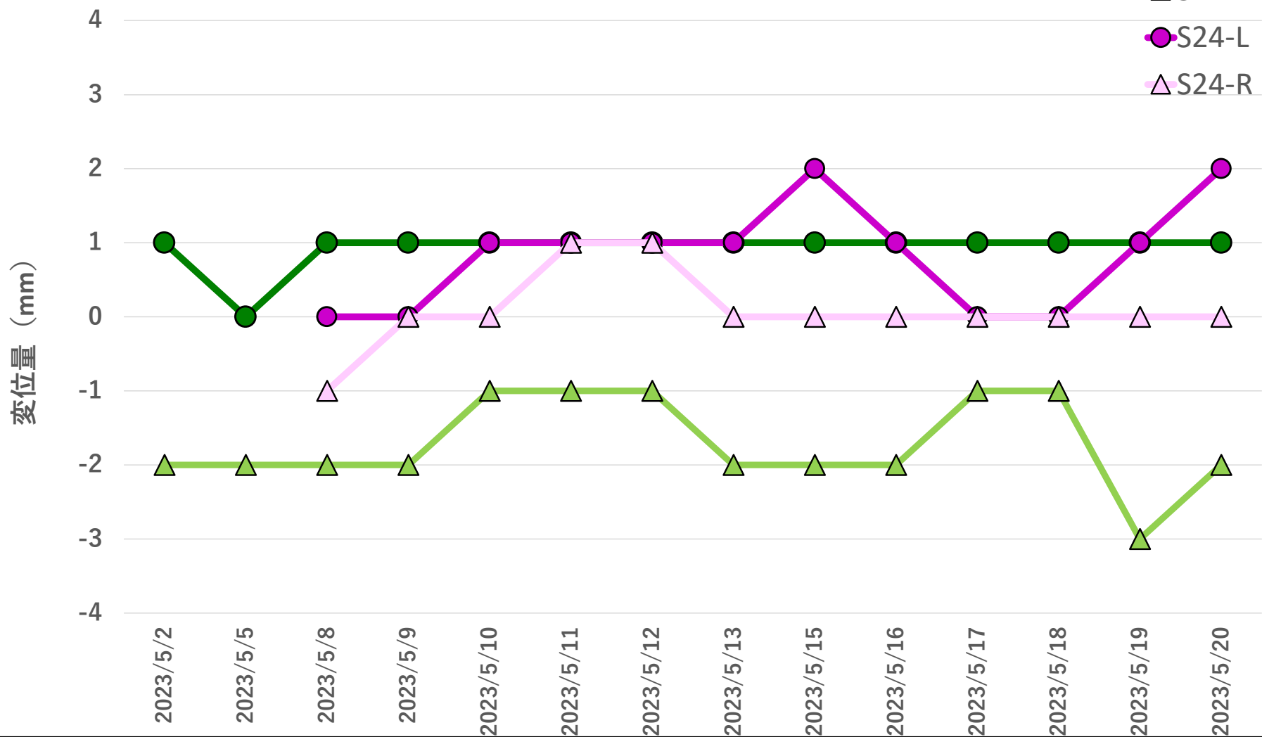
地盤変位量推移 2023年5月2日~2023年5月20日
