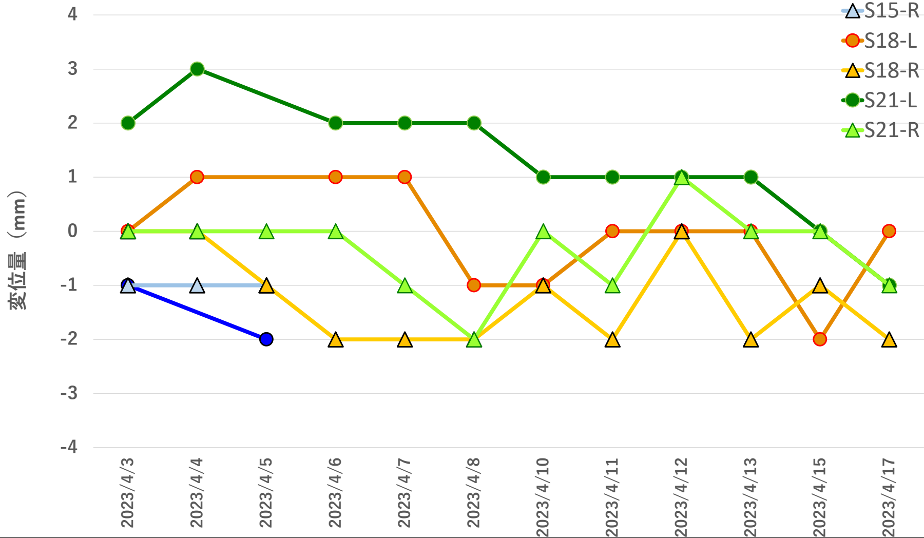
地盤変位量推移 2023年4月3日~2023年4月17日
