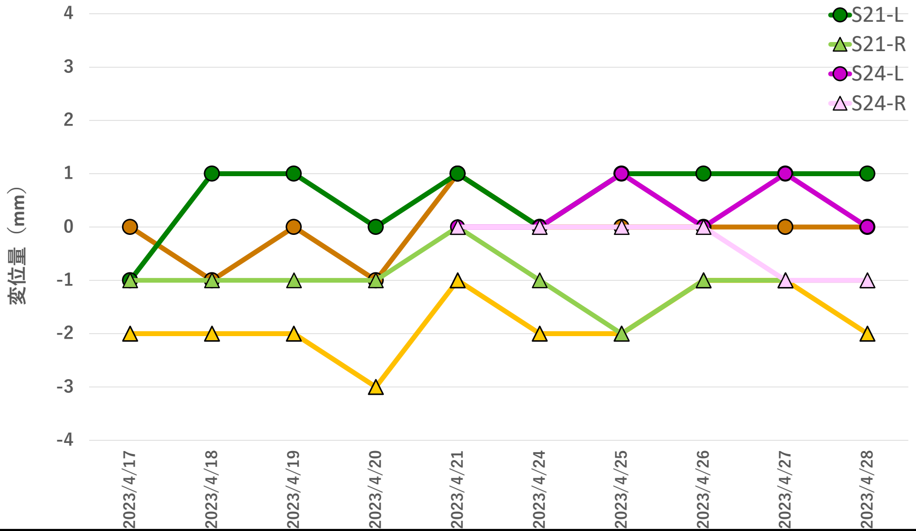
地盤変位量推移 2023年4月17日~2023年4月28日
