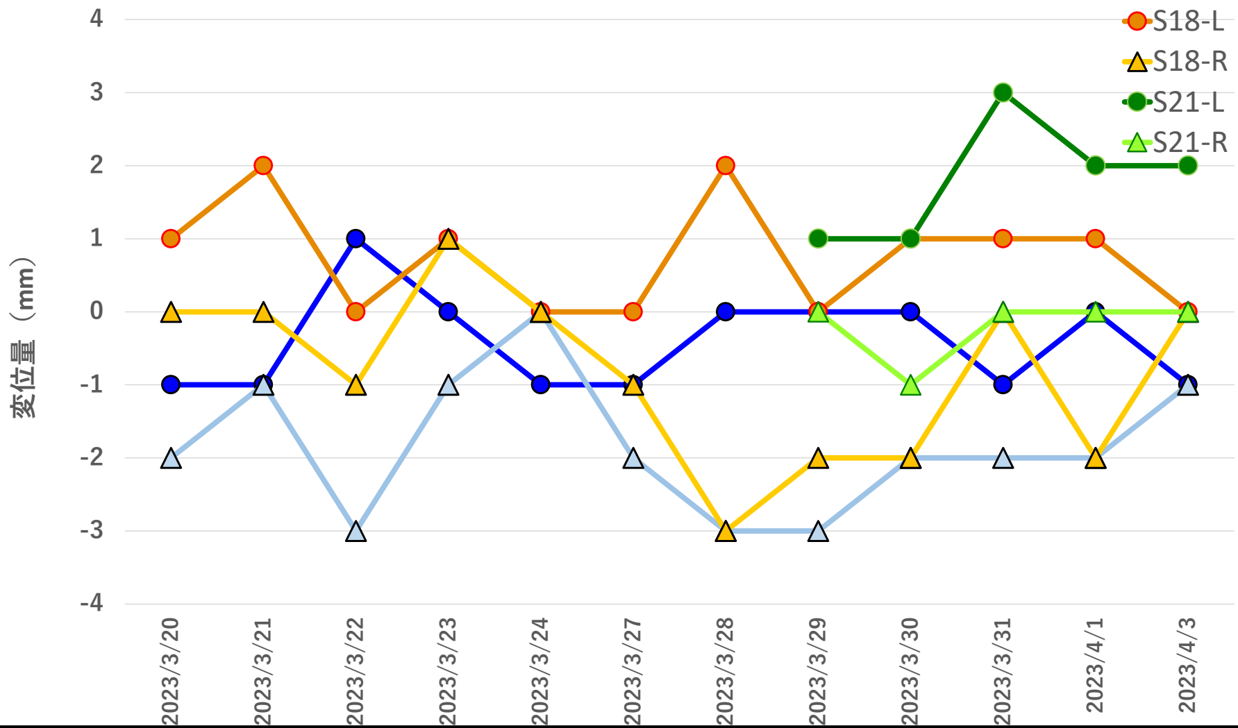
地盤変位量推移 2023年3月20日~2023年4月3日
